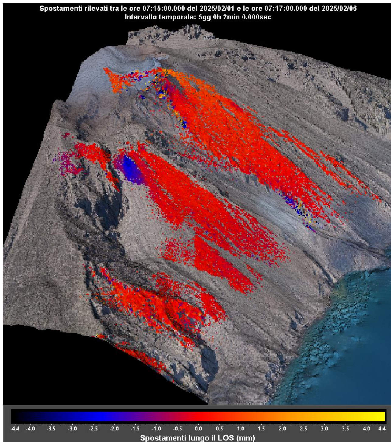
Figura 2 - Interferogramma registrato dal sistema GBInSAR NE190 riferito al tempo di 5 giorni e 2 minuti dalle ore 07:15 UTC (08:15 ora locale) del 01 febbraio 2025 alle ore 07:17 UTC (08:17 ora locale) del 06 febbraio 2025.
