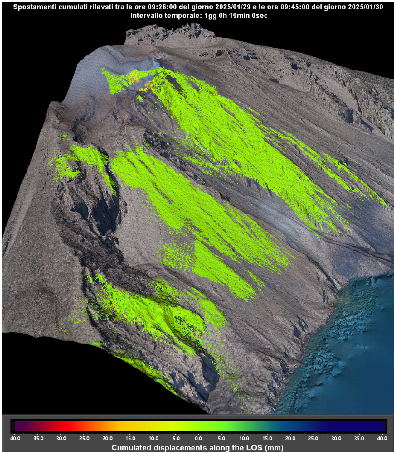
Figura 2 – Mappa cumulata delle deformazioni registrata dal sistema GBInSAR NE190 riferito al tempo di 1 giorno e 19 minuti dalle ore 09:26 UTC (10:26 ora locale) del 29 gennaio 2025 alle ore 09:45 UTC (10:45 ora locale) del 30 gennaio 2025.
