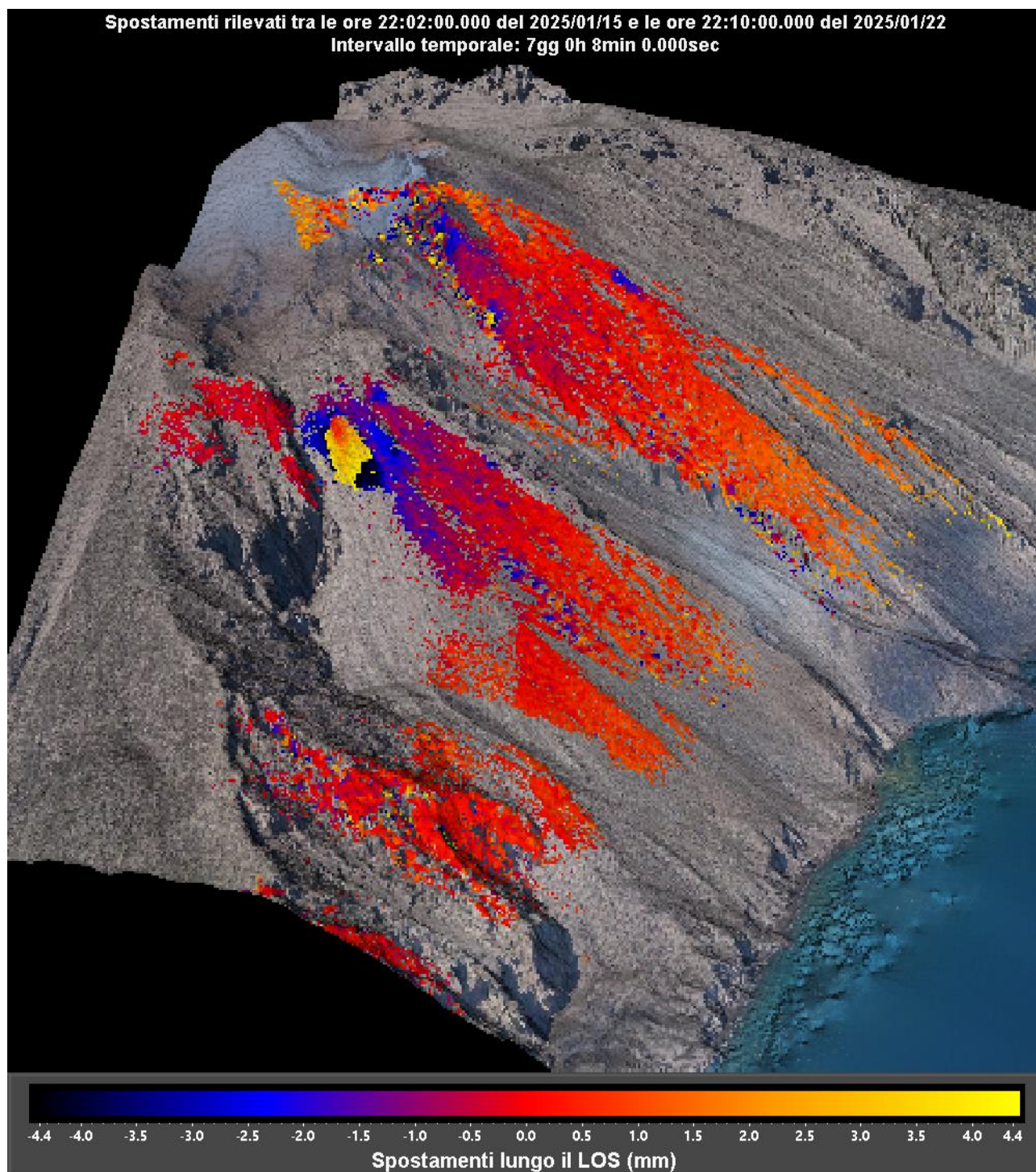
Figura 2 - Interferogramma registrato dal sistema GBInSAR NE190 riferito al tempo di 7 giorni e 8 minuti dalle ore 22:02 UTC (23:02 ora locale) del 15 gennaio 2025 alle ore 22:10 UTC (23:10 ora locale) del 22 gennaio 2025.
