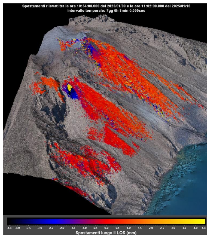
Figura 2 - Interferogramma registrato dal sistema GBInSAR NE190 riferito al tempo di 7 giorni e 8 minuti dalle ore 10:54 UTC (11:54 ora locale) del 09 gennaio 2025 alle ore 11:02 UTC (12:02 ora locale) del 16 gennaio 2025.
