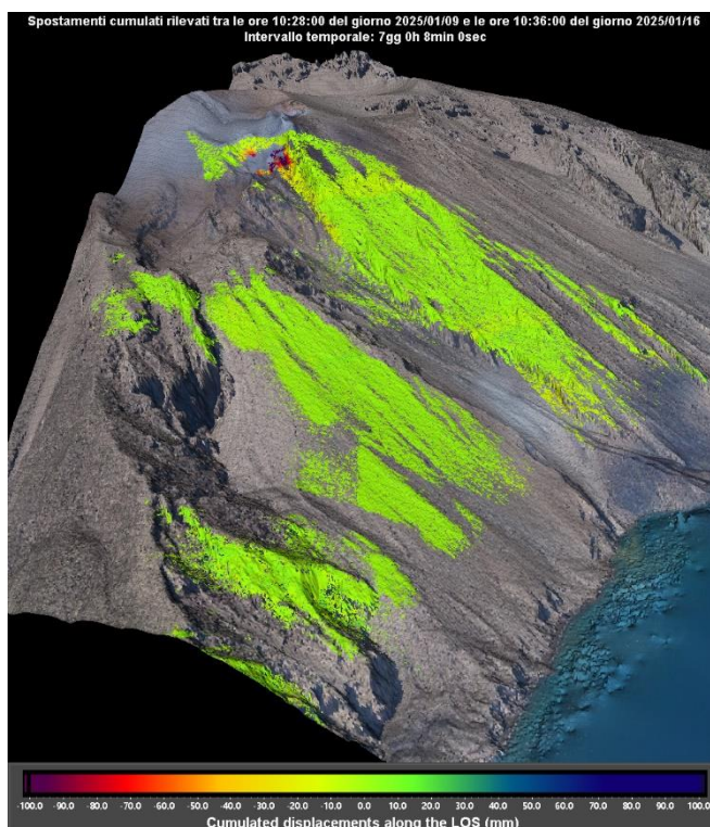
Figura 2 - Mappa cumulata delle deformazioni registrata dal sistema GBInSAR NE190 riferito al tempo di 7 giorni e 8 minuti dalle ore 10:28 UTC (11:28 ora locale) del 09 gennaio 2025 alle ore 10:36 UTC (11:36 ora locale) del 16 gennaio 2025.
