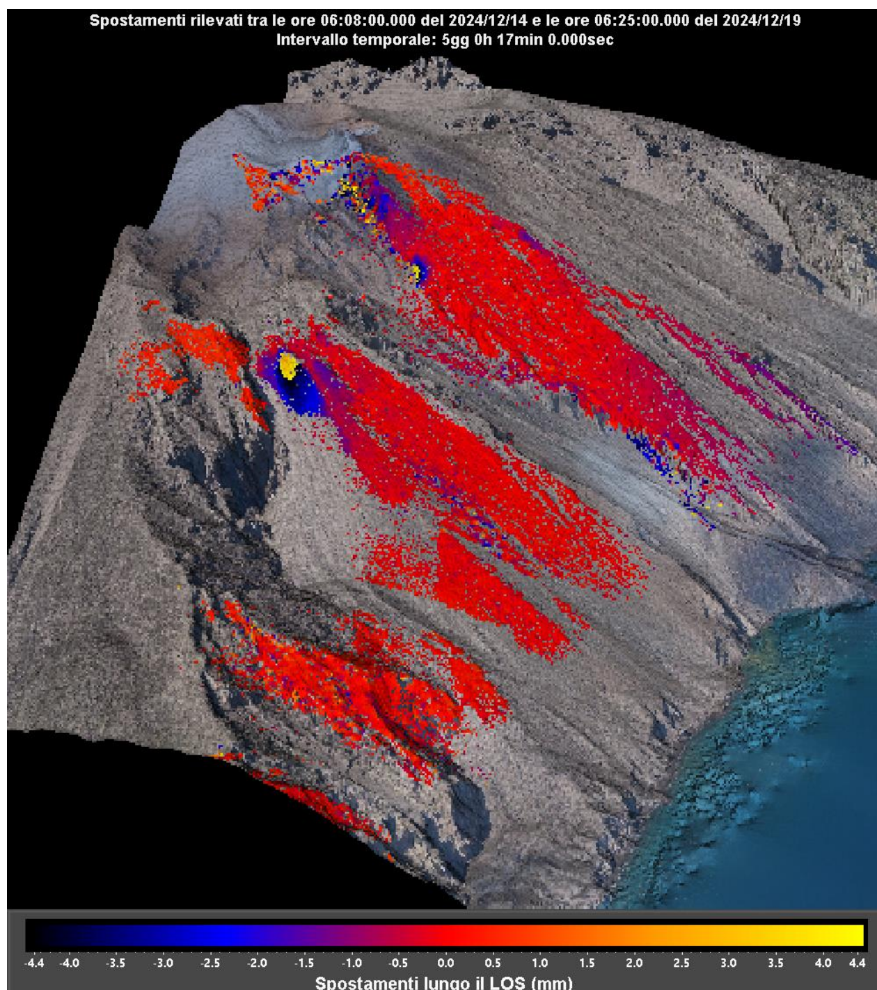
Figura 2 - Interferogramma registrato dal sistema GBInSAR NE190 riferito al tempo di 5 giorni e 17 minuti dalle ore 06:08 UTC (07:08 ora locale) del 14 dicembre 2024 alle ore 06:25 UTC (07:25 ora locale) del 19 dicembre 2024.
