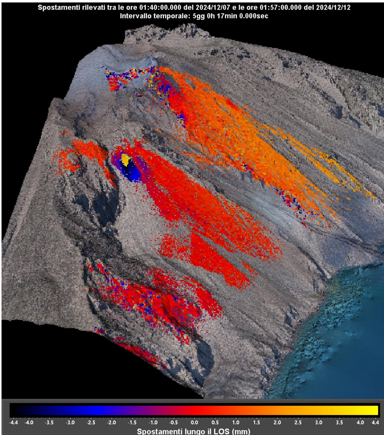
Figura 2 – Interferogramma registrato dal sistema GBInSAR NE190 riferito al tempo di 5 giorni dalle ore 01:40 UTC (02:40 ora locale) del 07 dicembre 2024 alle ore 01:57 UTC (02:57 ora locale) del 12 dicembre 2024.
