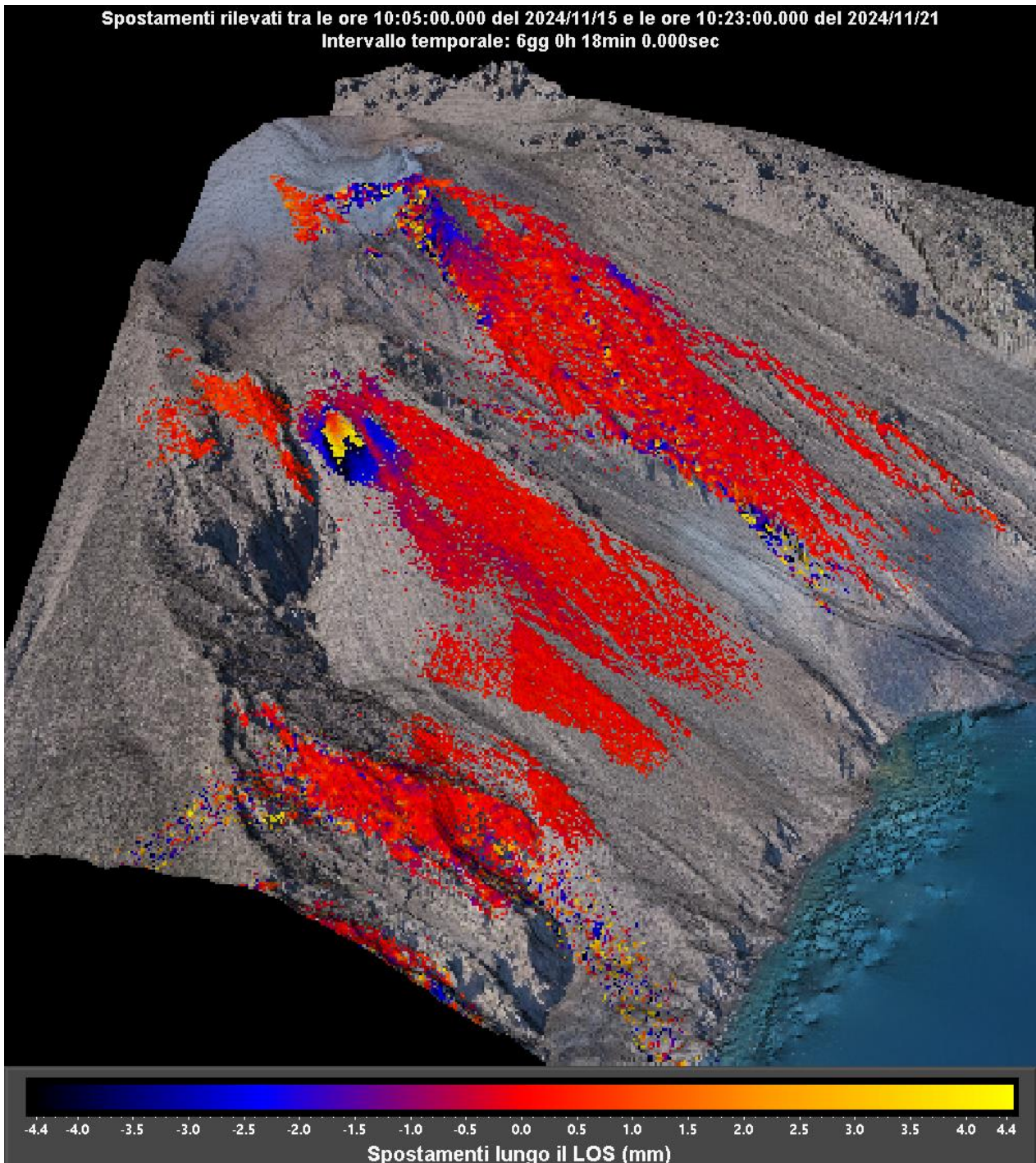
Figura 2 – Interferogramma registrato dal sistema GBInSAR NE190 riferito al tempo di 6 giorni e 18 minuti dalle ore 10:05 UTC (11:05 ora locale) del 15 novembre 2024 alle ore 10:23 UTC (11:23 ora locale) del 21 novembre 2024.
