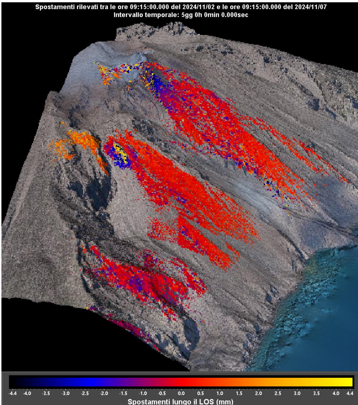
Figura 2 – Interferogramma registrato dal sistema GBInSAR NE190 riferito al tempo di 3 giorni e 22 minuti dalle ore 11:59 UTC (12:59 ora locale) del 27 ottobre 2024 alle ore 12:21 UTC (13:21 ora locale) del 30 ottobre 2024.
