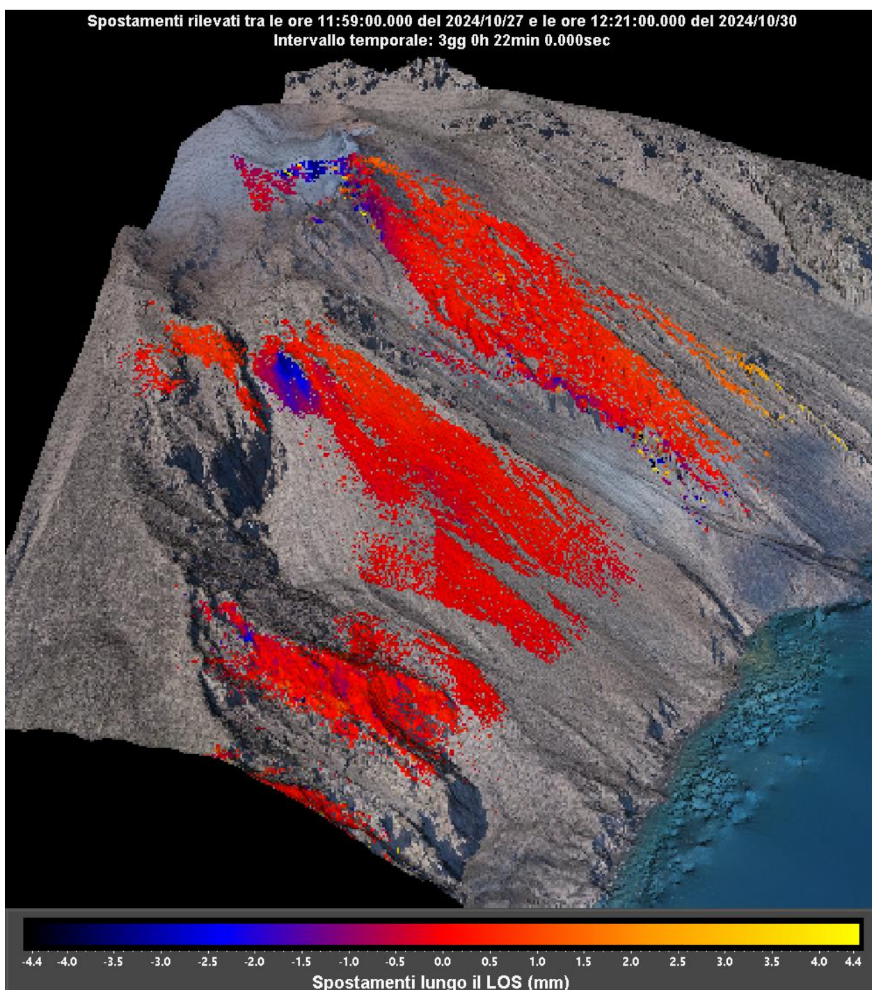
Figura 2 – Interferogramma registrato dal sistema GBInSAR NE190 riferito al tempo di 3 giorni e 22 minuti dalle ore 11:59 UTC (12:59 ora locale) del 27 ottobre 2024 alle ore 12:21 UTC (13:21 ora locale) del 30 ottobre 2024.
