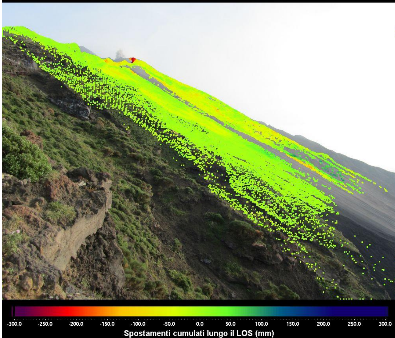
Figura 2 – Mappa cumulata delle deformazioni registrata dal sistema GBInSAR NE190 riferita al tempo di 30 giorni e 3 minuti dalle ore 09:29 UTC (10:29 ora locale) del 17 settembre 2024 alle ore 09:32 UTC (11:32 ora locale) del 17 ottobre 2024.
