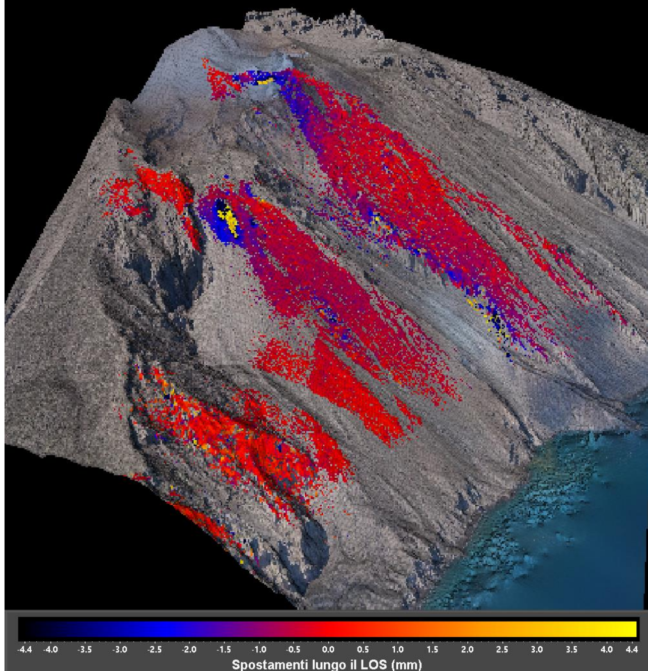
Figura 2 – Interferogramma registrato dal sistema GBInSAR NE190 riferito al tempo di 2 giorni e 24 minuti dalle ore 06:56 UTC (08:56 ora locale) del 24 settembre 2024 alle ore 07:20 UTC (09:20 ora locale) del 26 settembre 2024.
