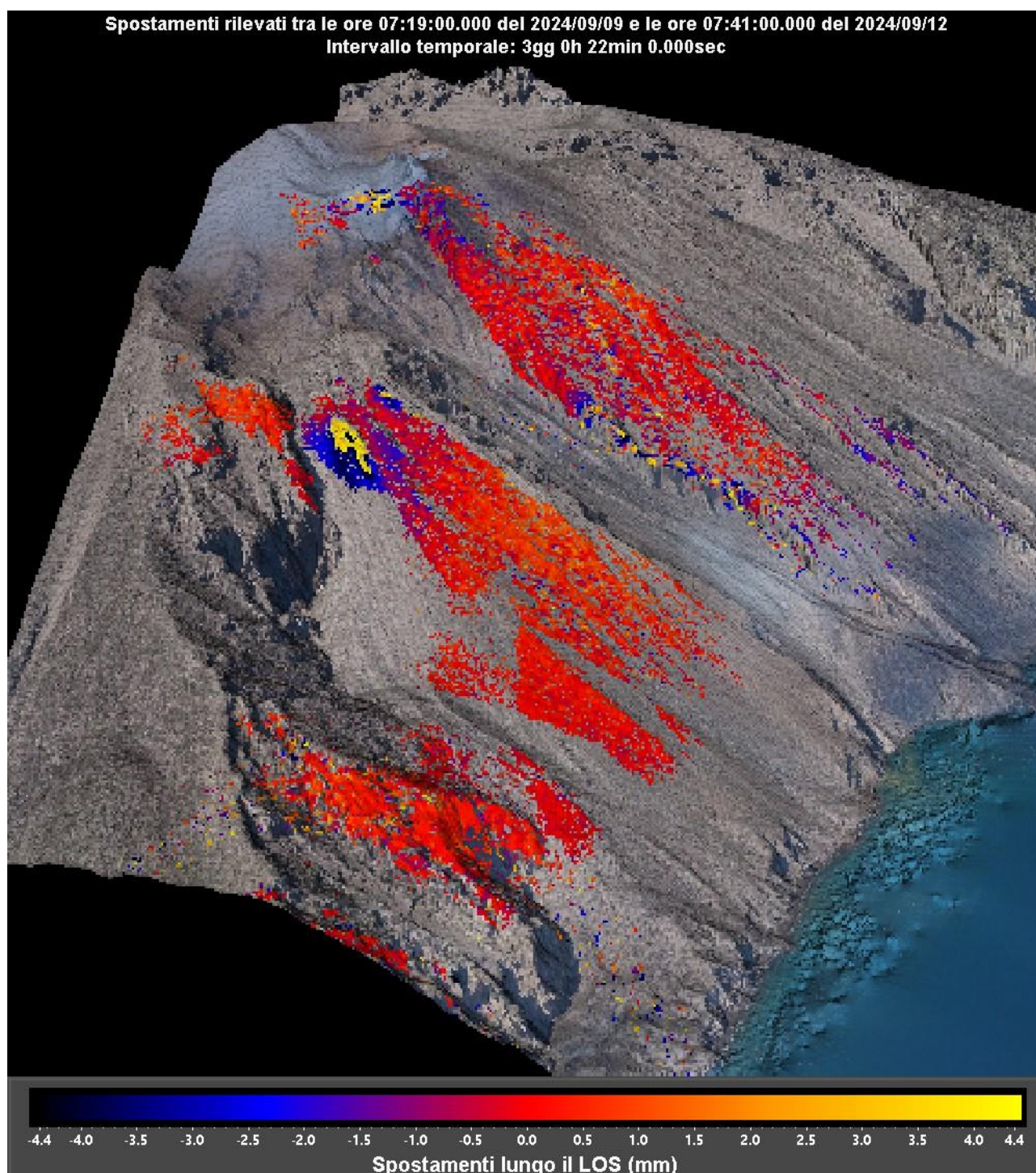
Figura 2 – Interferogramma registrato dal sistema GBInSAR NE190 riferito al tempo di 3 giorni e 22 minuti dalle ore 07:19 UTC (09:19 ora locale) del 09 settembre 2024 alle ore 07:41 UTC (09:41 ora locale) del 12 settembre 2024.
