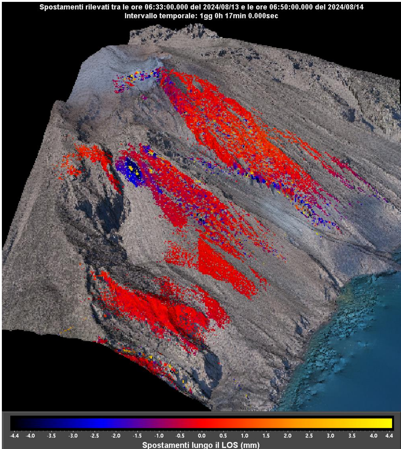
Figura 2 – Interferogramma registrato dal sistema GBInSAR NE190 riferito al tempo di 1 giorno e 17 minuti dalle ore 06:33 UTC (08:33 ora locale) del 13 agosto 2024 alle ore 06:50 UTC (08:50 ore locali) del 14 agosto 2024.
