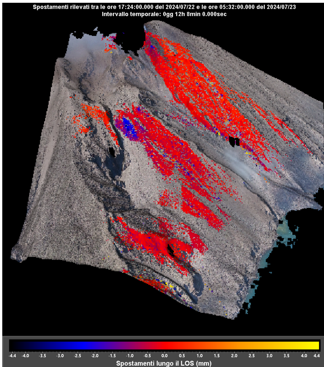
Figura 2 - Interferogramma registrato dal sistema GBInSAR NE190 riferito al tempo di 12 ore e 08 minuti dalle ore 17:24 UTC (19:24 ora locale) del 22 luglio 2024 alle ore 05:32 UTC (07:32 ore locali) del 23 luglio 2024.
