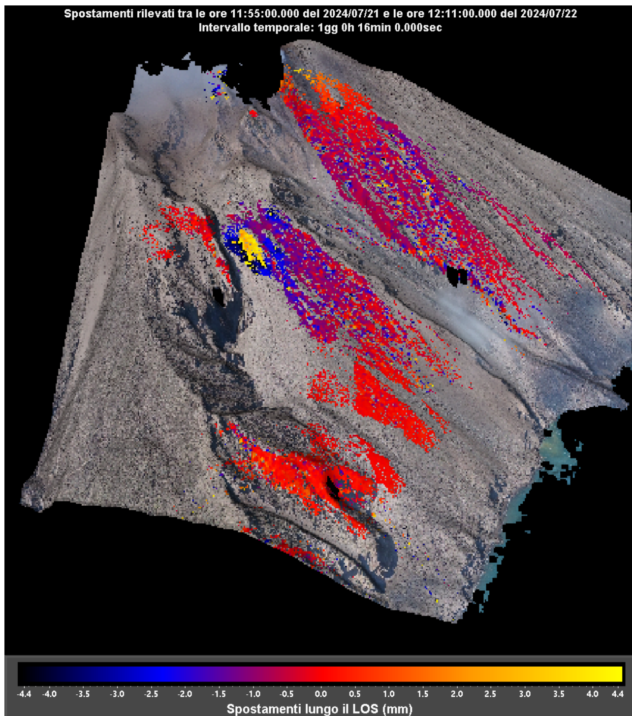
Figura 2 - Interferogramma registrato dal sistema GBInSAR NE190 riferito al tempo di 1 giorno e 16 minuti dalle ore 11:55 UTC (13:55 ora locale) del 21 luglio 2024 alle ore 12:11 UTC (14:11 ore locali) del 22 luglio 2024.
