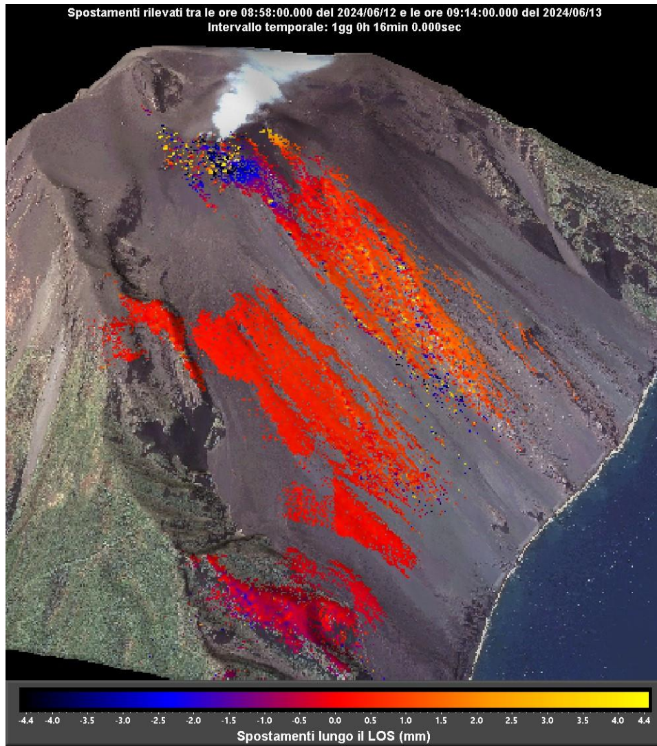
Figura 2 – Interferogramma registrato dal sistema GBInSAR NE190 riferito al tempo di 1 giorno e 16 minuti dalle ore 08:58 UTC (10:58 ora locale) del 12 giugno 2024 alle ore 09:14 UTC (10:14 ore locali) del 13 giugno 2024.
