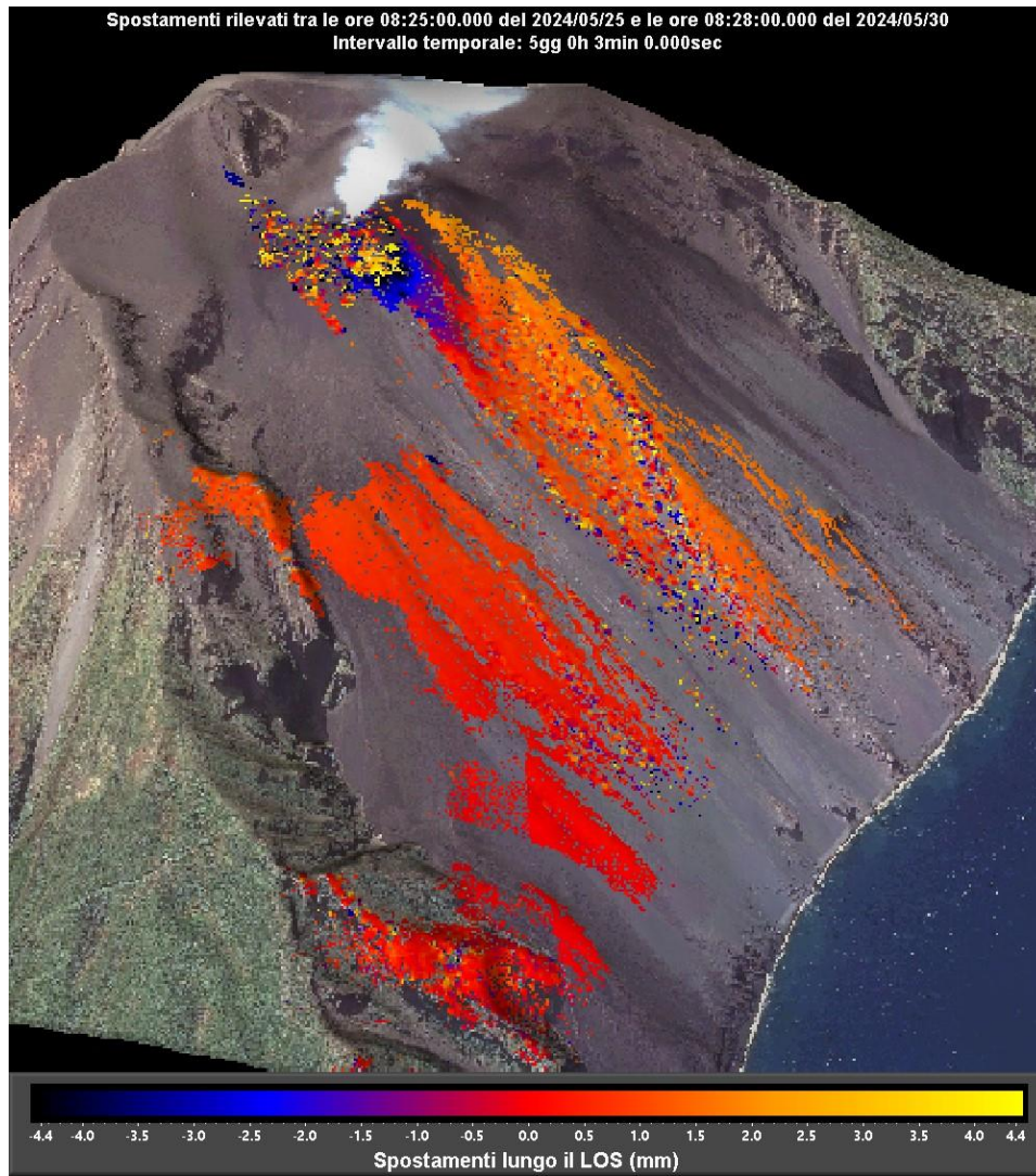
Figura 2 – Interferogramma registrato dal sistema GBInSAR NE190 riferito al tempo di 5 giorni e 7 minuti dalle ore 08:25 UTC (10:25 ora locale) del 25 maggio 2024 alle ore 08:28 UTC (10:28 ore locali) del 30 maggio 2024.
