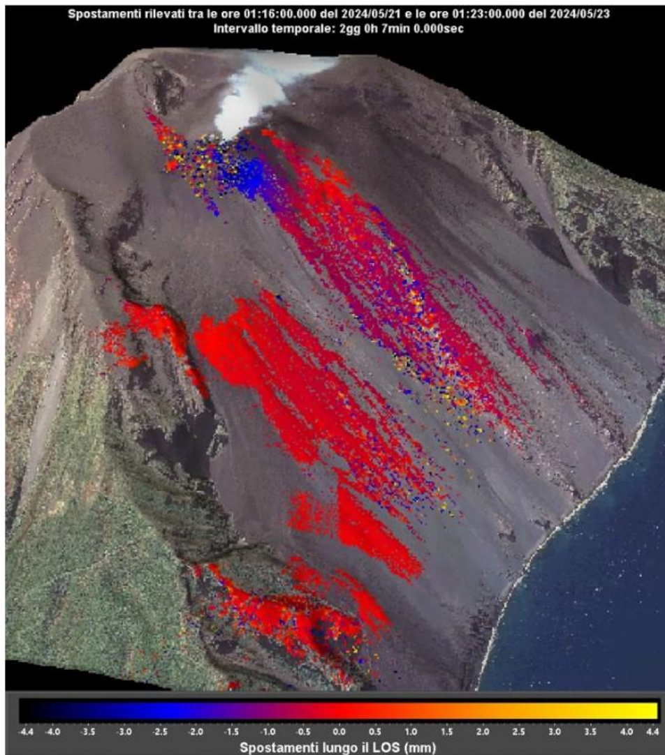
Figura 2 – Interferogramma registrato dal sistema GBInSAR NE190 riferito al tempo di 2 giorni e 7 minuti dalle ore 01:16 UTC (03:16 ora locale) del 21 maggio 2024 alle ore 01:23 UTC (03:23 ore locali) del 23 maggio 2024.
