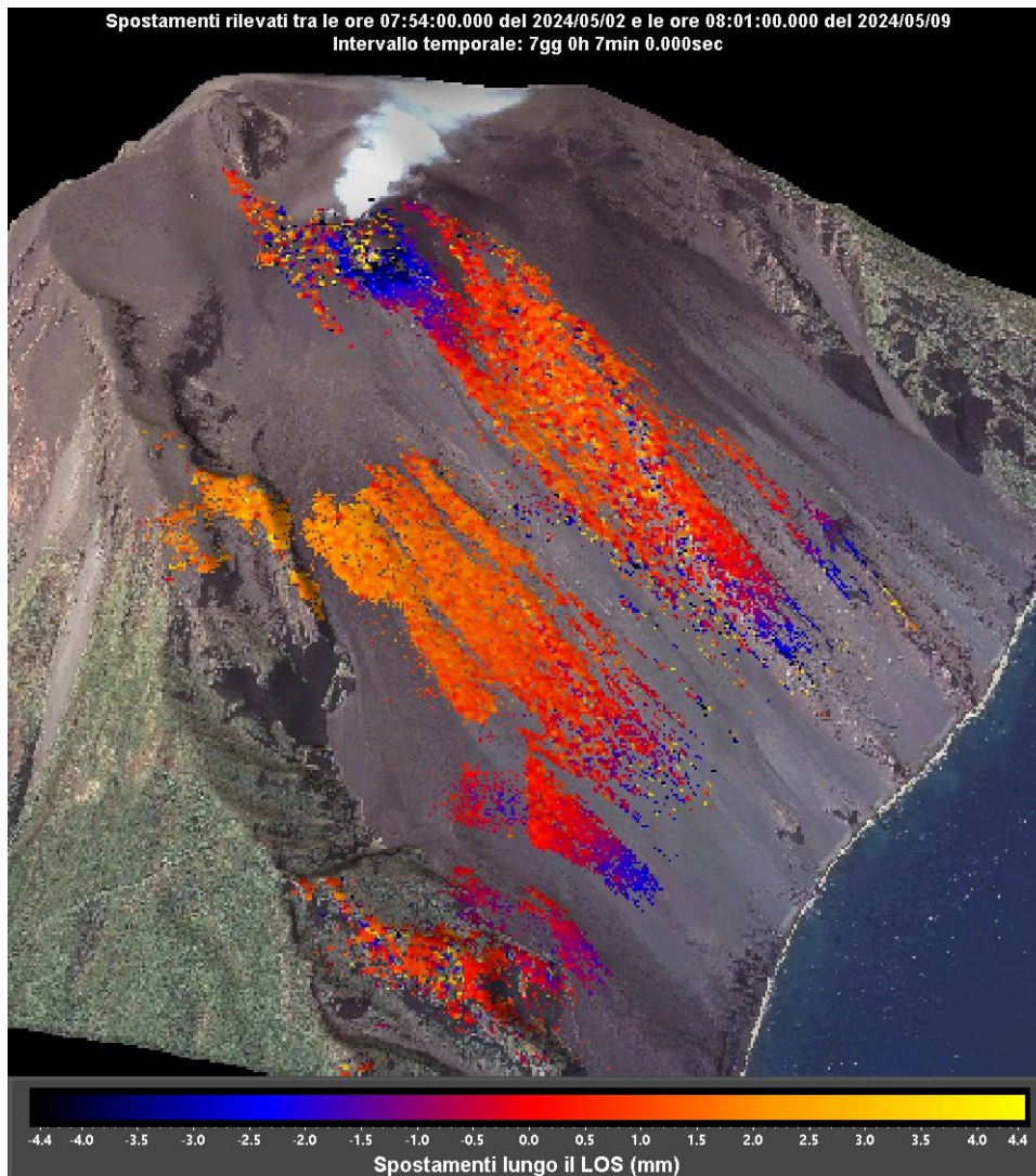
Figura 2 – Interferogramma registrato dal sistema GBInSAR NE190 riferito al tempo di 7 giorni e 7 minuti dalle ore 07:54 UTC (09:54 ora locale) del 02 maggio 2024 alle ore 08:01 UTC (10:01 ore locali) del 07 maggio 2024.
