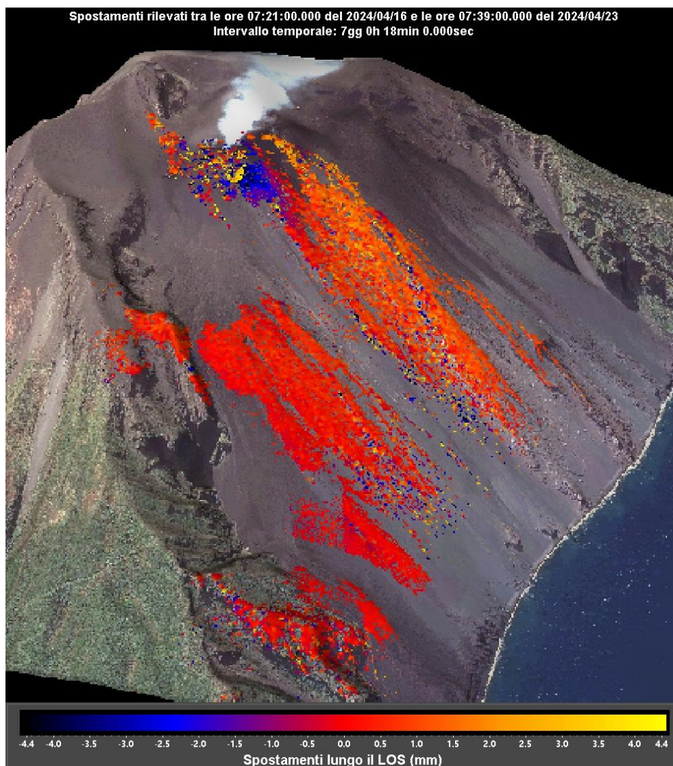
Figura 2 – Interferogramma registrato dal sistema GBInSAR NE190 riferito al tempo di 7 giorni e 18 minuti dalle ore 07:21 UTC (09:21 ora locale) del 16 aprile 2024 alle ore 07:39 UTC (9:39 ore locali) del 23 aprile 2024.
