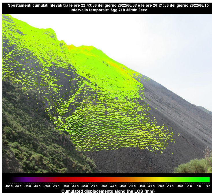
Figura 2 - Mappa degli spostamenti cumulati registrata dal sistema GBInSAR NE400 riferita al tempo di 6 giorni 21 ore e 38 minuti dalle ore 22:43 UTC del 08 giugno 2022 (00:43 ora locale del 09 giugno 2022) alle ore 20:21 UTC (22:21 ore locali) del 15 giugno 2022.
