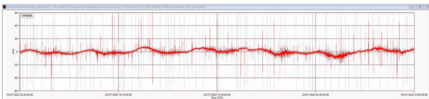
Fig. 13.1 Segnale gravimetrico registrato nella stazione VFARA dalle 22:00 UTC del 18 alle 22:00 UTC del 25 luglio 2022. In grigio il segnale acquisito al secondo; la traccia colorata indica il segnale mediato al minuto. I segnali sono corretti per gli effetti della marea terrestre e della deriva strumentale.
