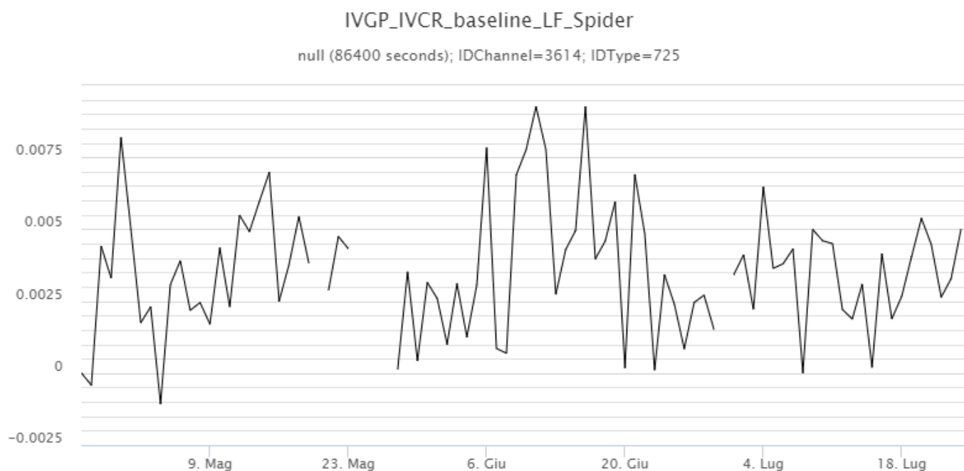
Fig. 11.1 Serie temporale a bassa frequenza (1 dato al giorno) della variazione di distanza IVGP-IVCR
