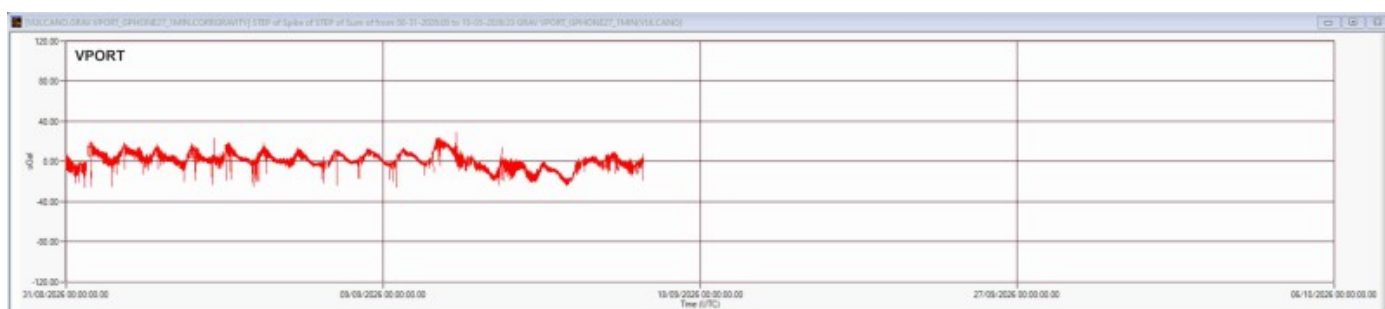
Fig. 13.1 Segnale gravimetrico registrato nella stazione VPORT dalle 00:00 UTC del 31 agosto 2026 alle 09:30 UTC del 16 settembre 2026. Il segnale è mediato al minuto. I dati sono corretti per gli effetti della marea terrestre e della deriva strumentale.
