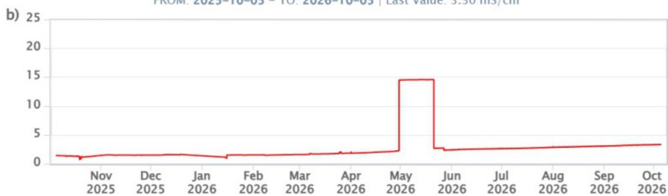
Fig. 8.1 Dati di temperatura e conducibilità riferita a 20°C, acquisiti in automatico nel pozzo Camping Sicilia.
