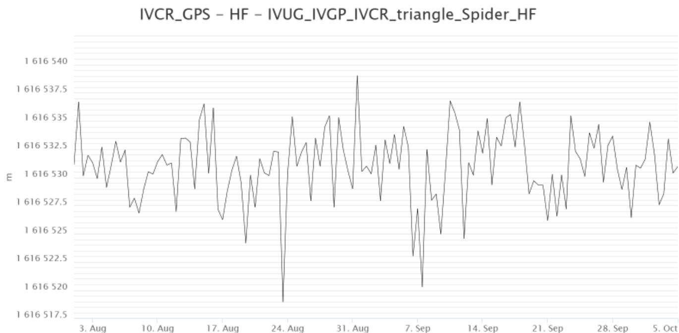
Fig. 11.1 Dilatazione areale del triangolo IVCR-IVGP-IVUG
