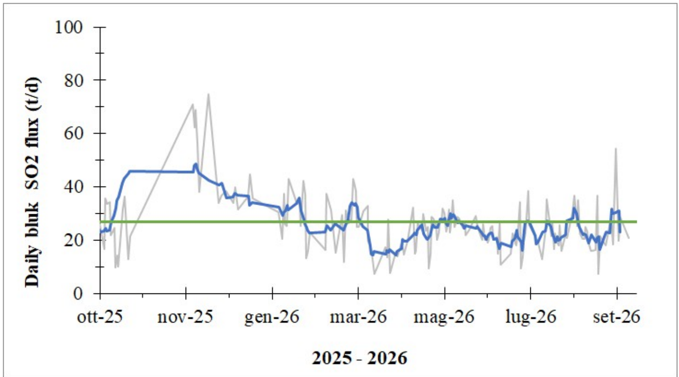
Fig. 5.1 Il flusso di SO 2 medio-giornaliero e medio-settimanale emesso dal campo fumarolico craterico di Vulcano nell'ultimo anno (rispettivamente, linea grigia e blu)
