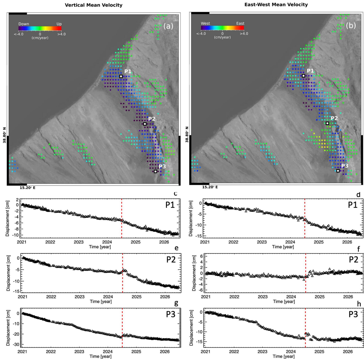
Figura 2. Mappe delle componenti Verticale ed Est-Ovest della velocità media di deformazione dell'area settentrionale della Sciara del Fuoco relative al periodo 24 aprile 2015 – 26 giugno 2026. a) Componente Verticale. b) Componente Est-Ovest. c-h) Andamento temporale della deformazione lungo la direzione Verticale (c)(e)(g) ed Est-Ovest (d)(f)(h) in corrispondenza di tre punti identificati come P1a, P1b e P1c in (a)-(b) nel periodo gennaio 2021 – 26 giugno 2026. La linea rossa tratteggiata indica gli eventi di inizio luglio 2024.
