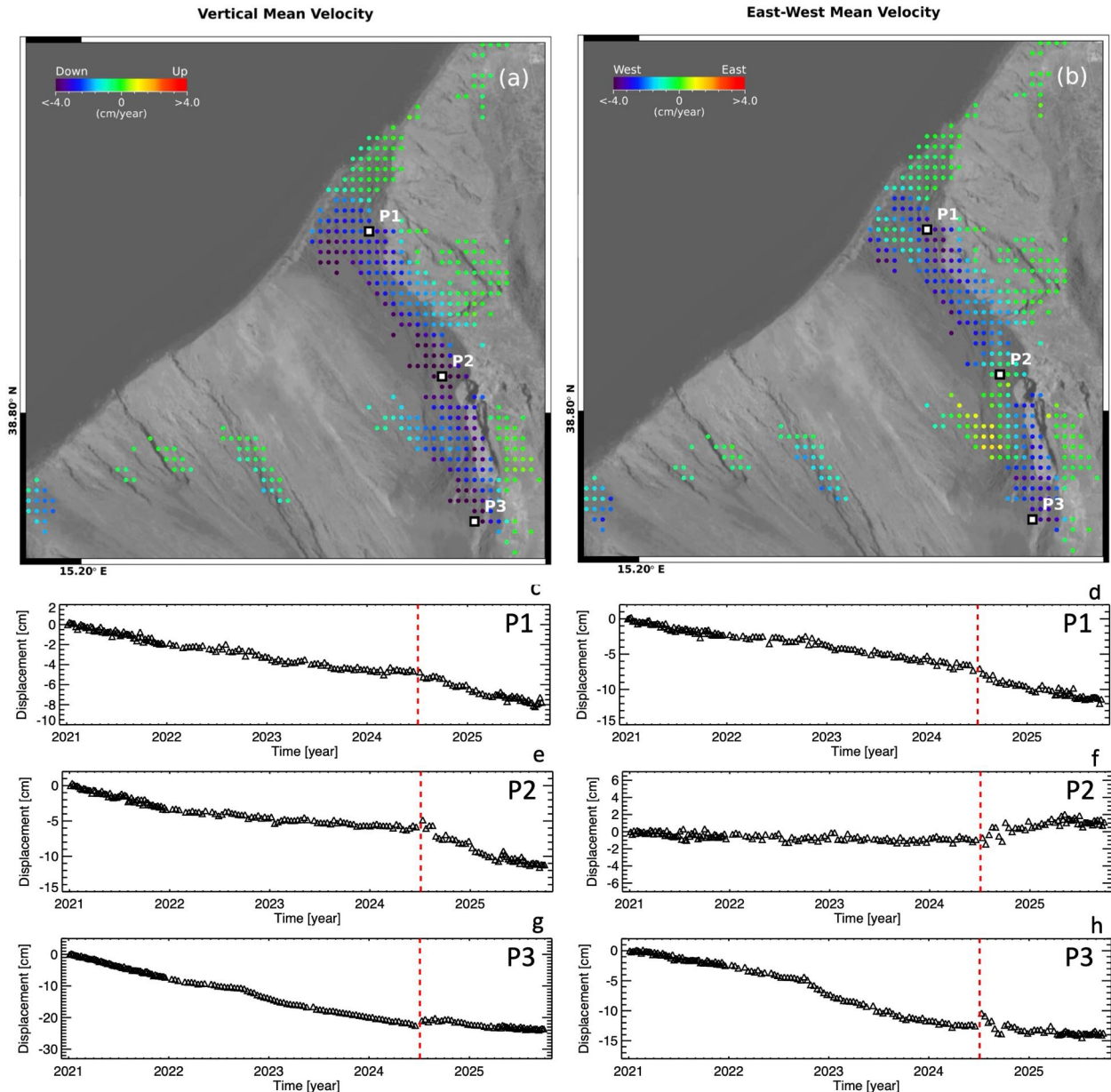
Figura 2. Mappe delle componenti Verticale ed Est-Ovest della velocità media di deformazione dell'area settentrionale della Sciara del Fuoco relative al periodo 24 aprile 2015 – 28 settembre 2025. a) Componente Verticale. b) Componente Est-Ovest. c-h) Andamento temporale della deformazione lungo la direzione Verticale (c)(e)(g) ed Est-Ovest (d)(f)(h) in corrispondenza di tre punti identificati come P1a, P1b e P1c in (a)-(b) nel periodo gennaio 2021 – 28 settembre 2025. La linea rossa tratteggiata indica gli eventi di inizio luglio 2024.
