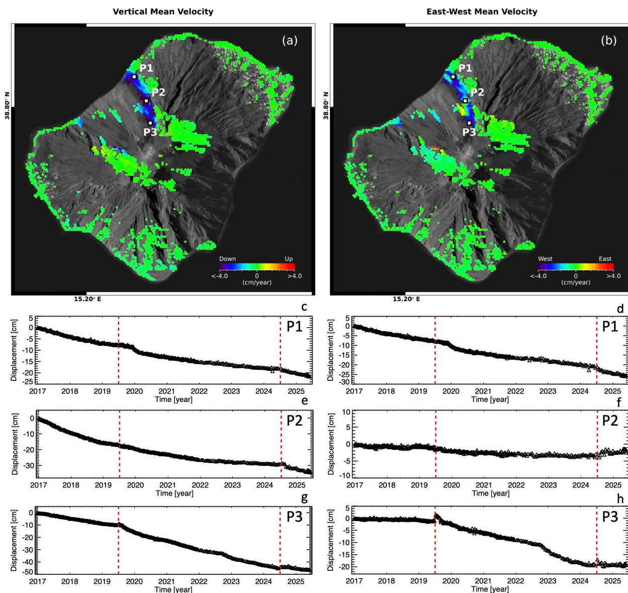
Figura 1. Mappe delle componenti Verticale ed Est-Ovest della velocità media di deformazione relative al periodo 24 aprile 2015 – 31 maggio 2025 generate a partire da dati Sentinel-1. a) Componente Verticale. b) Componente Est-Ovest. c-h) Andamento temporale della deformazione lungo la direzione Verticale (c)(e)(g) ed Est-Ovest (d)(f)(h) in corrispondenza di tre punti identificati come P1, P2 e P3 in (a)-(b) nel periodo gennaio 2017 – 31 maggio 2025. Le linee rosse tratteggiate indicano il parossismo del 3 luglio 2019 e gli eventi di inizio luglio 2024.
