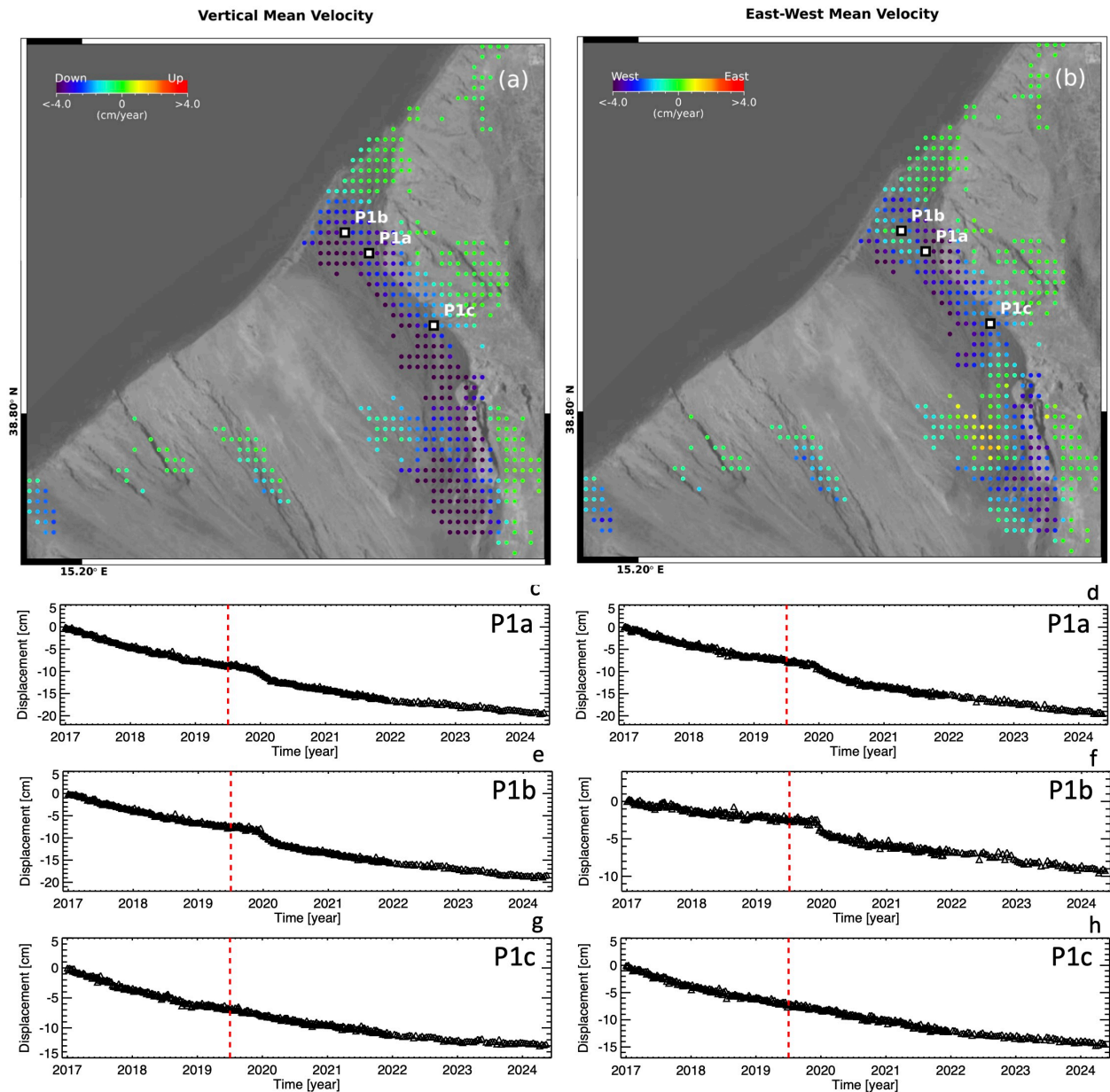
Figura 2. Mappe delle componenti Verticale ed Est-Ovest della velocità media di deformazione dell'area settentrionale della Sciara del Fuoco relative al periodo 24 aprile 2015 – 24 maggio 2024. a) Componente Verticale. b) Componente Est-Ovest. c-h) Andamento temporale della deformazione lungo la direzione Verticale (c)(e)(g) ed Est-Ovest (d)(f)(h) in corrispondenza di tre punti identificati come P1a, P1b e P1c in (a)-(b) nel periodo gennaio 2017 – 24 maggio 2024. La linea rossa tratteggiata indica il parossismo del 3 luglio 2019.
