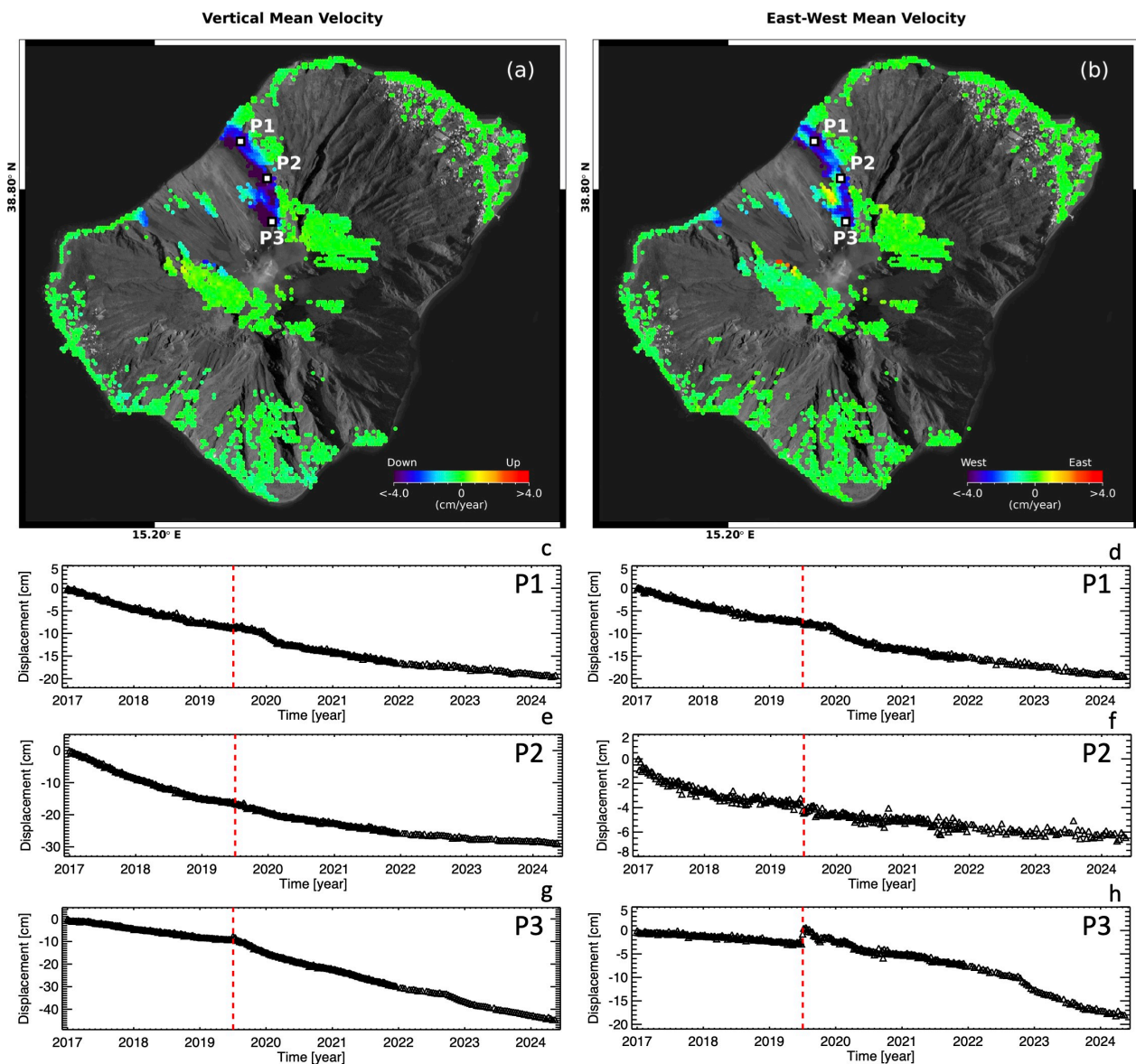
Figura 1. Mappe delle componenti Verticale ed Est-Ovest della velocità media di deformazione relative al periodo 24 aprile 2015 – 24 maggio 2024 generate a partire da dati Sentinel-1. a) Componente Verticale. b) Componente Est-Ovest. c-h) Andamento temporale della deformazione lungo la direzione Verticale (c)(e)(g) ed Est-Ovest (d)(f)(h) in corrispondenza di tre punti identificati come P1, P2 e P3 in (a)-(b) nel periodo gennaio 2017 – 24 maggio 2024. La linea rossa tratteggiata indica il parossismo del 3 luglio 2019.
