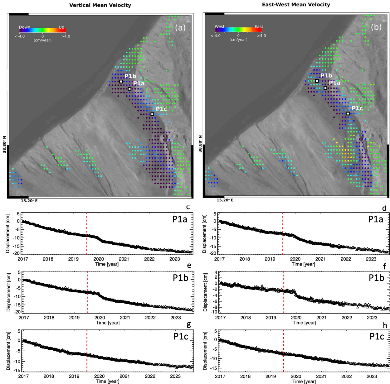
Figura 2. Mappe delle componenti Verticale ed Est-Ovest della velocità media di deformazione dell'area settentrionale della Sciara del Fuoco relative al periodo 24 aprile 2015 – 28 agosto 2023. a) Componente Verticale. b) Componente Est-Ovest. c-h) Andamento temporale della deformazione lungo la direzione Verticale (c)(e)(g) ed Est-Ovest (d)(f)(h) in corrispondenza di tre punti identificati come P1a, P1b e P1c in (a)-(b) nel periodo gennaio 2017 – 28 agosto 2023. La linea rossa tratteggiata indica il parossismo del 3 luglio 2019.
