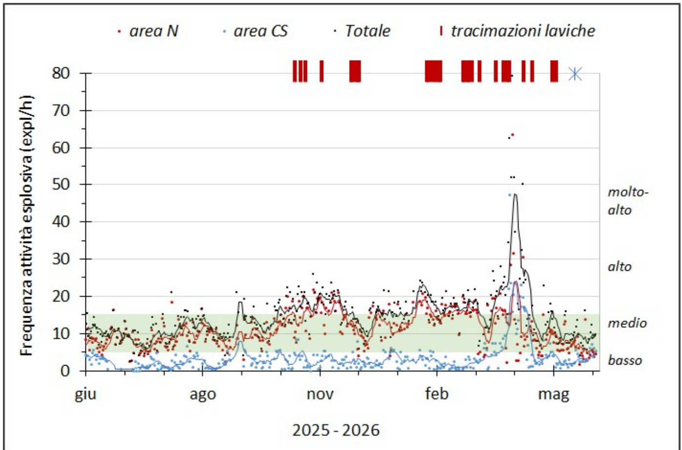
Fig. 3.2 Frequenza media oraria settimanale dell'attività esplosiva dello Stromboli, suddivisa per aree crateriche e totale (in rosso, azzurro e nero, rispettivamente). Nella parte superiore del grafico sono riportati gli episodi di attività effusiva da tracimazioni laviche dalle Aree Crateriche. La barra verde indica l'intervallo dei valori medi tipici dell'attività esplosiva. L'asterisco azzurro colloca l'esplosione maggiore del 12 giugno 2026.
