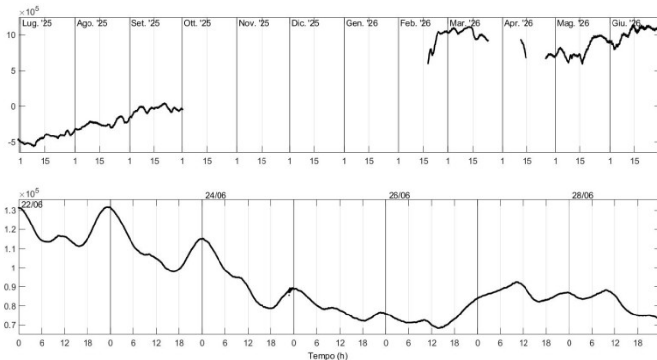
Fig. 4.3 Grafico relativo al dato dilatometrico registrato a SVO: in alto viene mostrato lo strain registrato nell'ultimo anno dal 30/06/2025; in basso quello registrato nell'ultima settimana.
