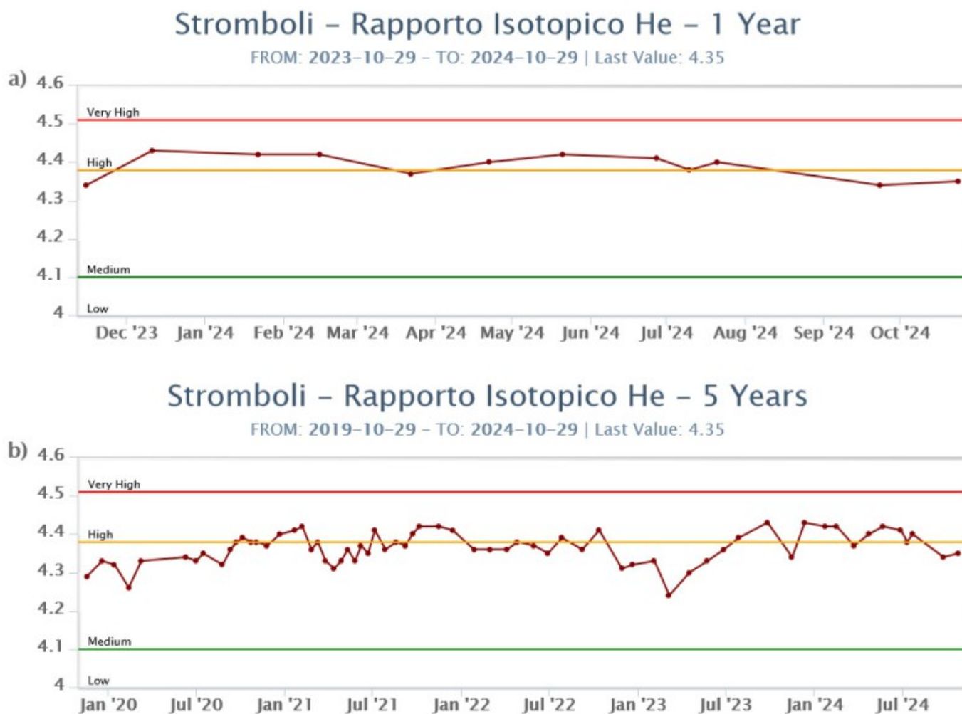
Fig. 6.4 Rapporto isotopico dell'He disciolto nei pozzi termali a) ultimo anno, b) ultimi 5 anni
