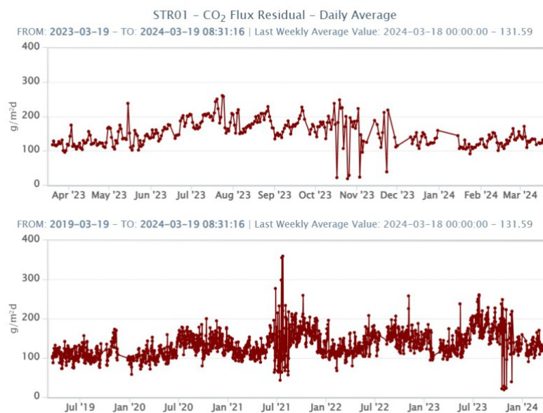
Fig. 6.5 Flussi di CO 2 dal suolo misurati in STR01 a) nell'ultimo anno; b) negli ultimi 5 anni.
