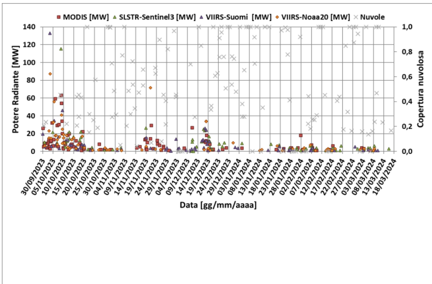
Fig. 7.1 Potere radiante calcolato da dati MODIS (quadrato rosso), SENTINEL-3 SLSTR (triangolo verde) e VIIRS (triangolo viola e rombo giallo) dal 30 settembre 2023 al 18 marzo 2024. Per l'intero periodo analizzato è anche riportato l'indice di nuvolosità.
