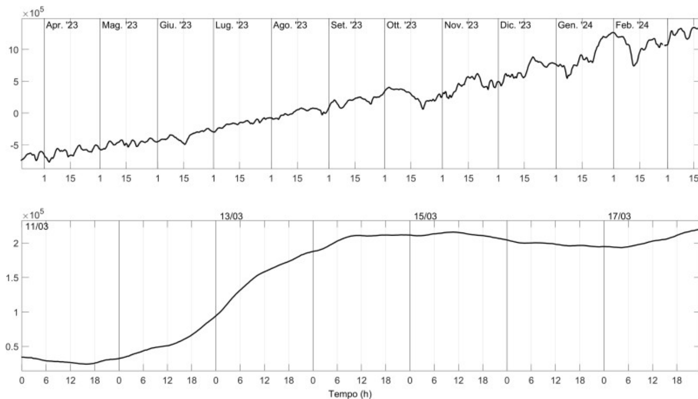
Fig. 4.3 Grafico relativo al dato dilatometrico registrato a SVO: in alto viene mostrato lo strain registrato dal 20/03/2023, in basso quello nell'ultima settimana.
