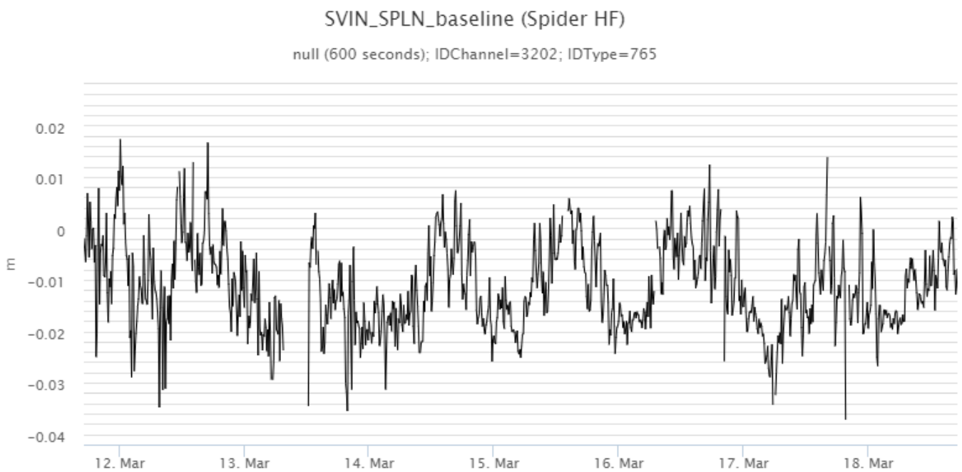
Fig. 5.2 Variazione di distanza tra le stazioni SVIN e SPLN
