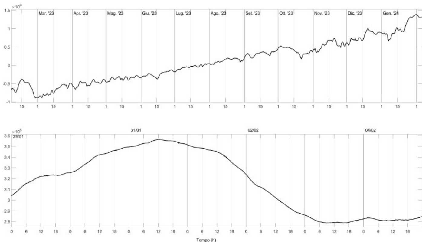
Fig. 4.3 Grafico relativo al dato dilatometrico registrato a SVO: in alto viene mostrato lo strain registrato dal 06/02/2023, in basso quello nell'ultima settimana.
