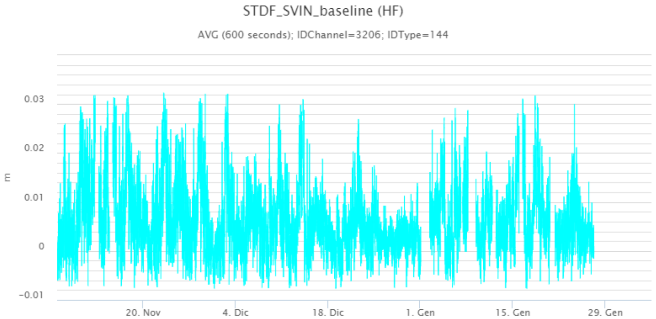
Fig. 5.1 Serie temporale della variazione di distanza (in m) tra le stazioni GNSS di SVIN e di STDF, nel corso dell'ultimo trimestre fino al 27 gennaio (nessun nuovo dato disponibile per la settimana in corso).
