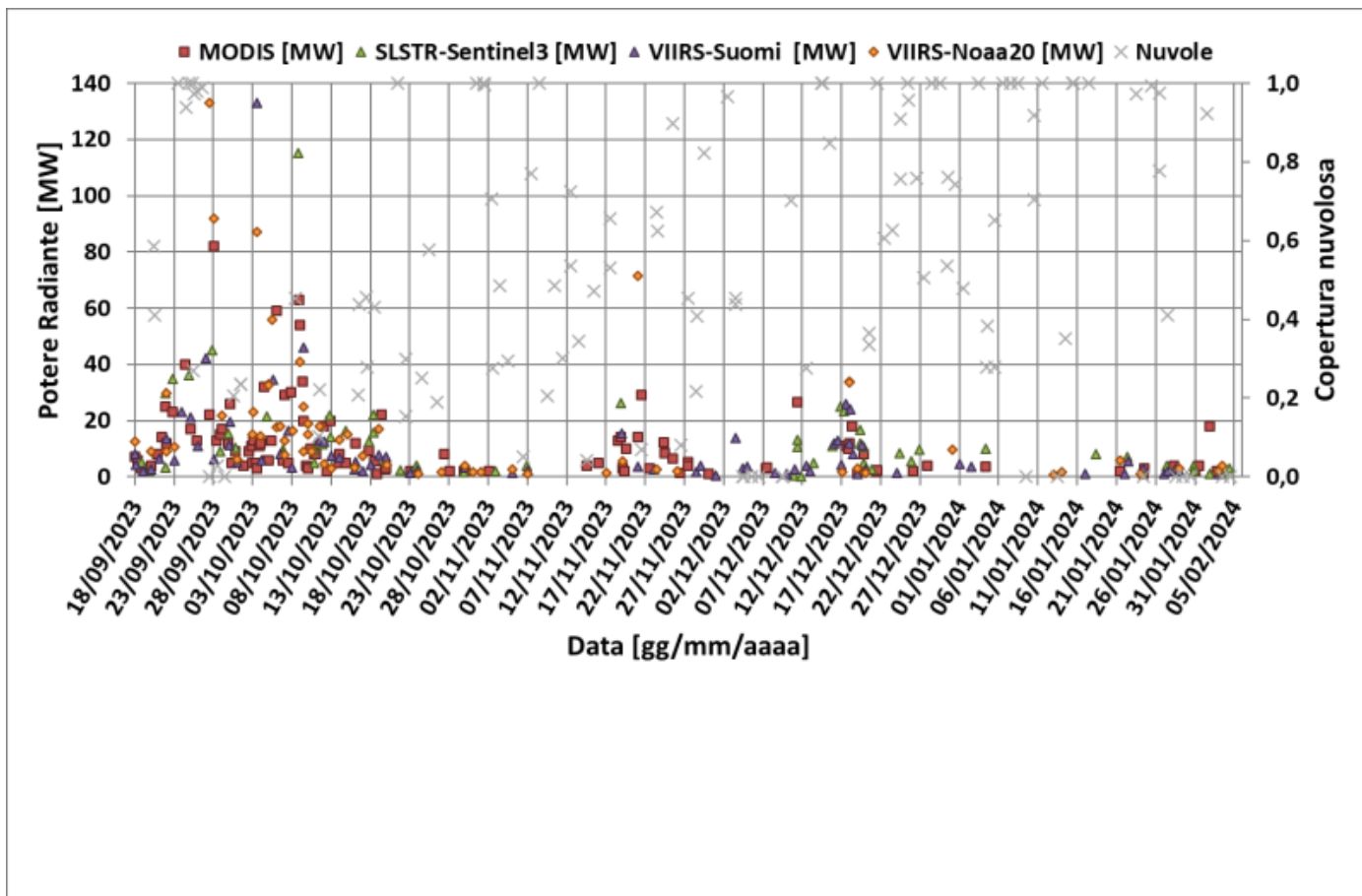
Fig. 7.1 Potere radiante calcolato da dati MODIS (quadrato rosso), SENTINEL-3 SLSTR (triangolo verde) e VIIRS (triangolo viola e rombo giallo) dal 18 settembre 2023 al 5 febbraio 2024. Per l'intero periodo analizzato è anche riportato l'indice di nuvolosità.
