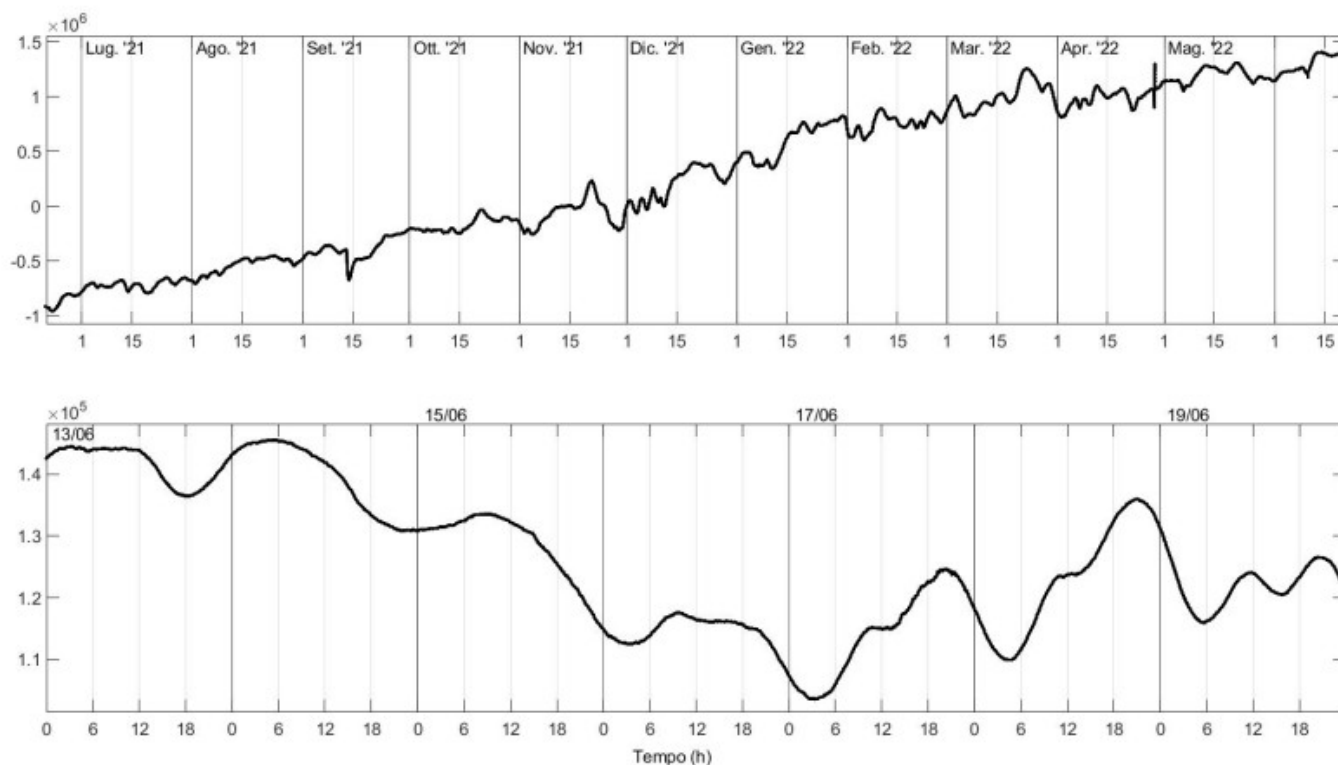
Fig. 4.4 Grafico relativo al dato dilatometrico registrato a SVO: in alto viene mostrato lo strain registrato dal 21/06/2021, in basso a sinistra quello nell'ultima settimana.
