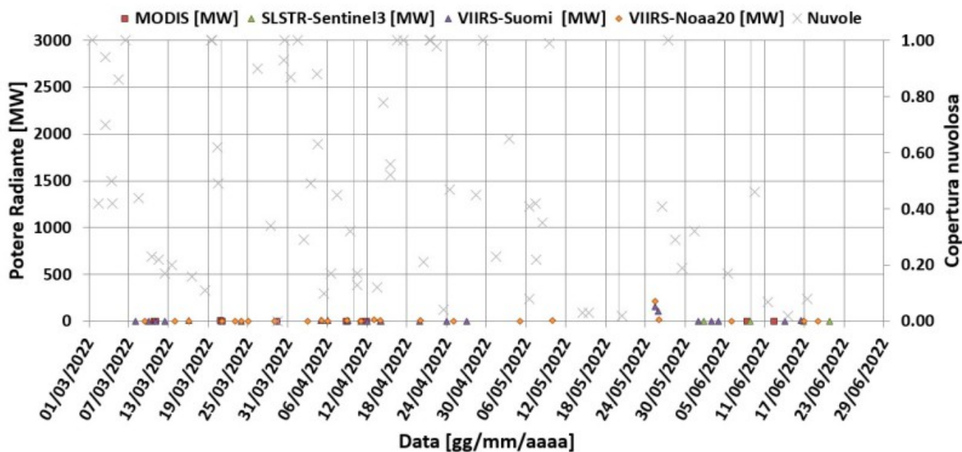
Fig. 7.1 Potere radiante calcolato da dati MODIS (quadrato rosso), SENTINEL-3 (triangolo verde) e VIIRS (triangolo viola e rombo giallo) dal primo marzo al 20 giugno 2022. Per l'intero periodo analizzato è anche riportato l'indice di nuvolosità.
