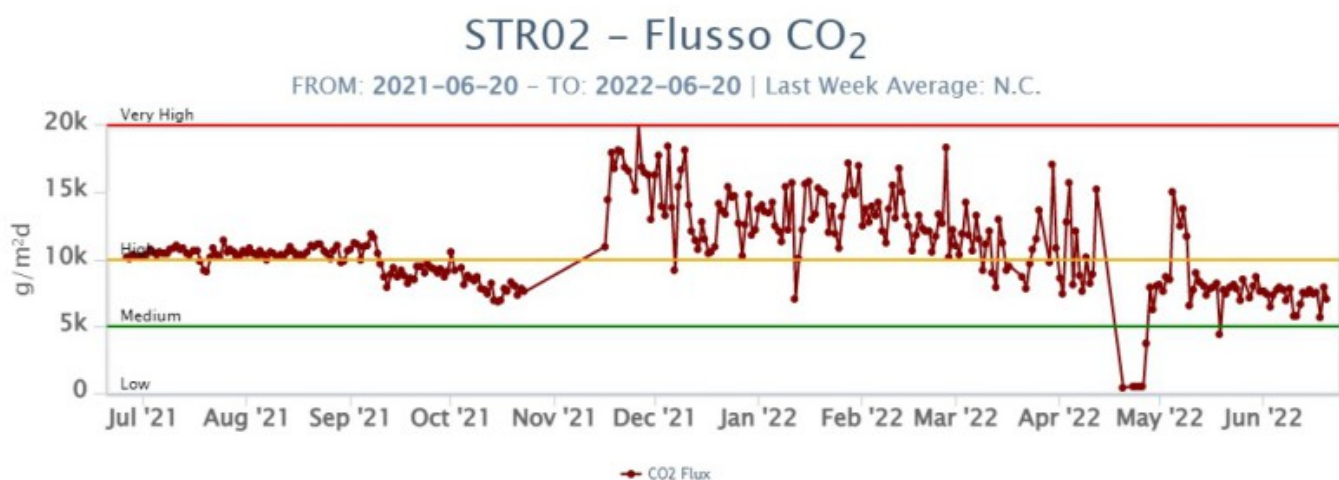
Fig. 6.2 Andamento temporale del flusso di CO 2 dal suolo in area sommitale (stazione STR02).
