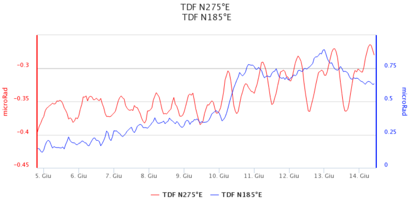
Fig. 5.2 Serie temporale delle componenti N275E e N185E [microradianti] della stazione clinometrica di TDF .
