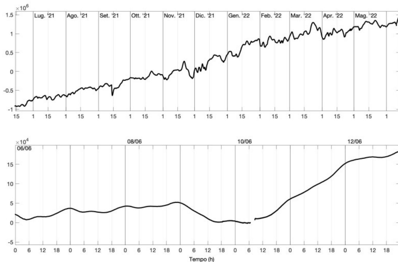
Fig. 4.4 Grafico relativo al dato dilatometrico registrato a SVO: in alto viene mostrato lo strain registrato dal 14/06/2021, in basso a sinistra quello nell'ultima settimana.
