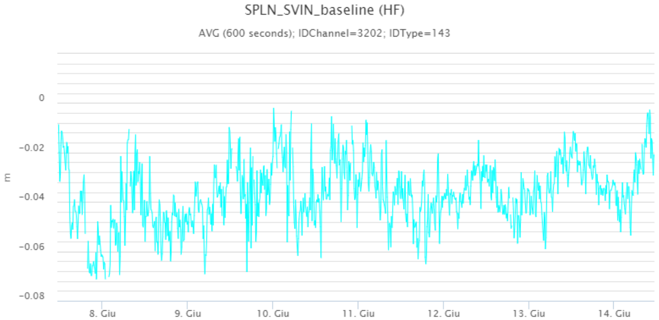
Fig. 5.1 Serie temporale della variazione di distanza [m] tra le stazioni GNSS di SVIN e di SPLN
