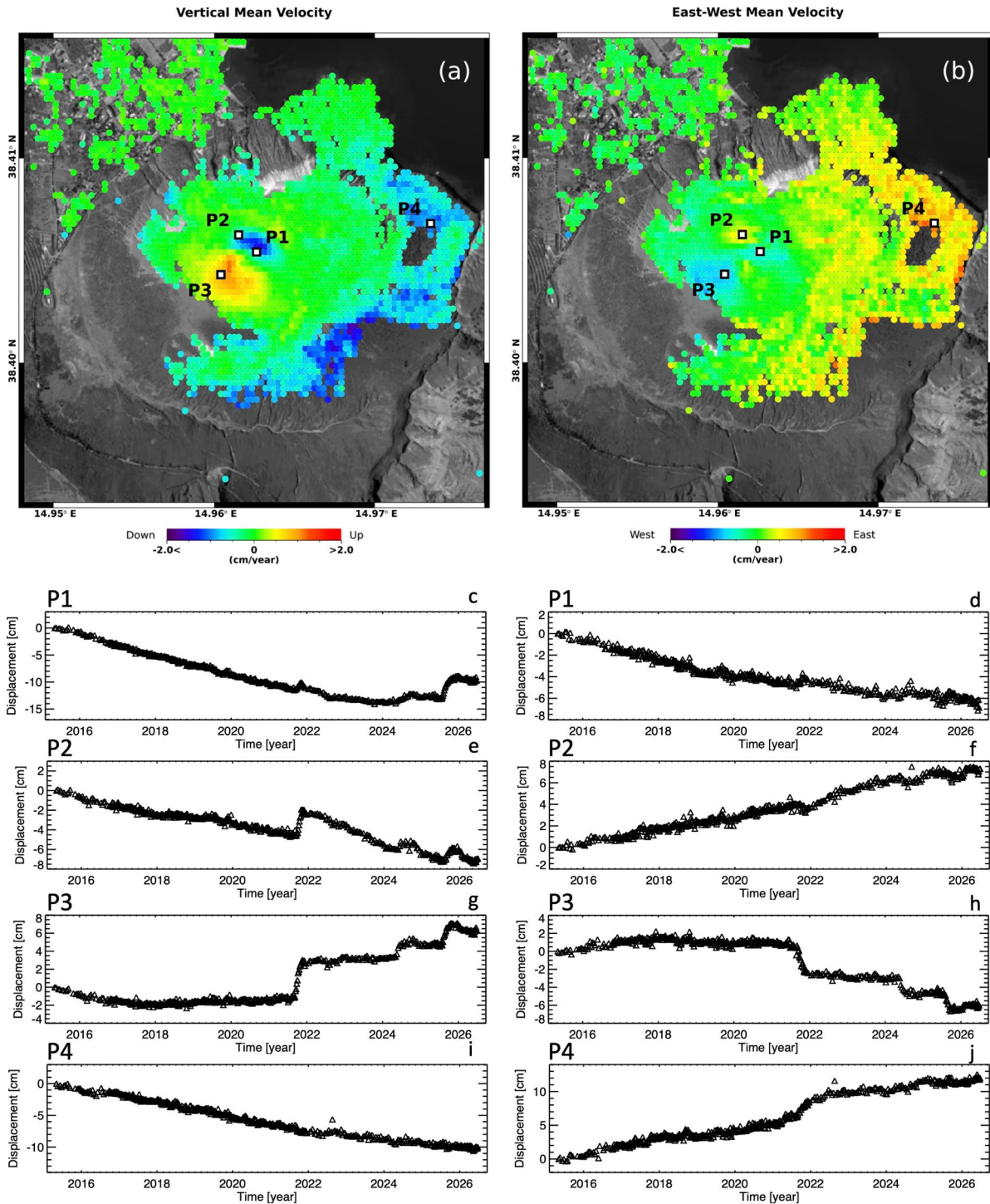
Figura 2. Vulcano – La Fossa: mappe delle componenti Verticale ed Est-Ovest della velocità media di deformazione relative al periodo 24 aprile 2015 – 26 giugno 2026 generate a partire da dati Sentinel-1. a) Componente Verticale. b) Componente Est-Ovest. c-j) Andamento temporale della deformazione lungo la direzione Verticale (c)(e)(g)(i) ed Est-Ovest (d)(f)(h)(j) in corrispondenza di quattro punti identificati come P1, P2, P3 e P4 in (a)-(b).
