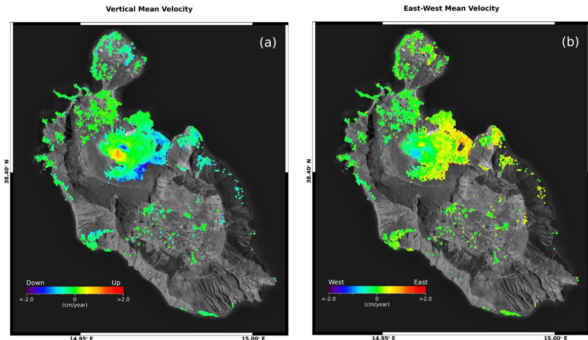
Figura 1. Vulcano: mappe delle componenti Verticale ed Est-Ovest della velocità media di deformazione relative al periodo 24 aprile 2015 – 26 giugno 2026 generate a partire da dati Sentinel-1. a) Componente Verticale. b) Componente Est-Ovest.
