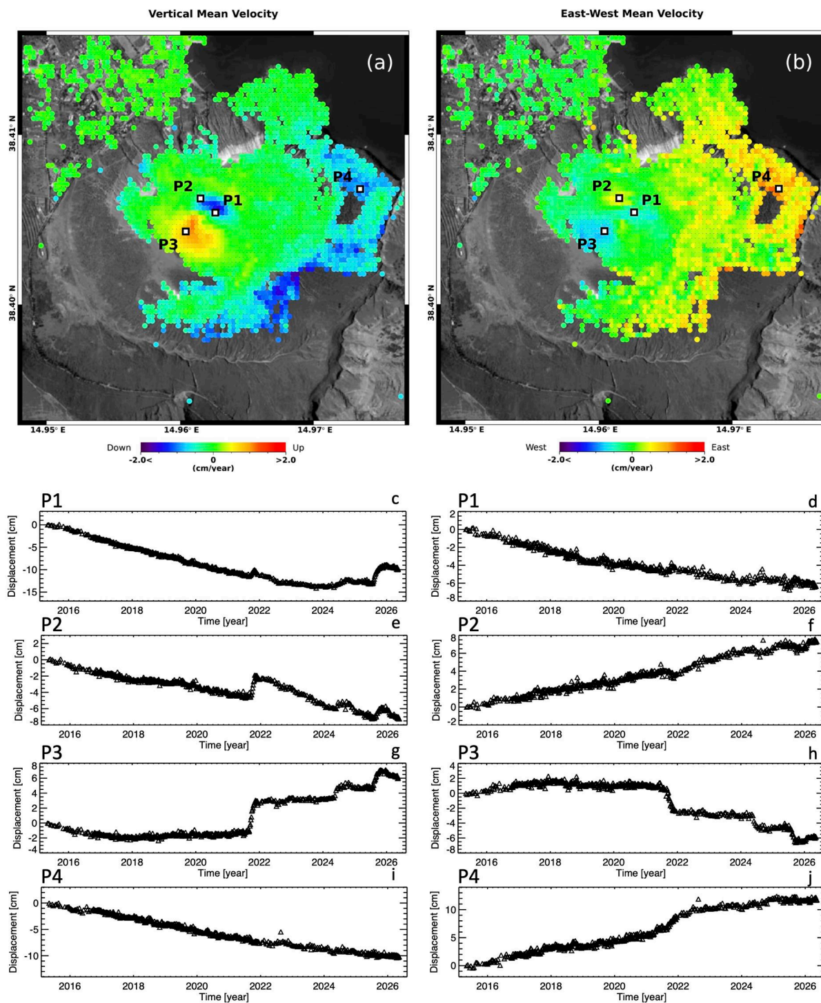
Figura 2. Vulcano – La Fossa: mappe delle componenti Verticale ed Est-Ovest della velocità media di deformazione relative al periodo 24 aprile 2015 – 14 maggio 2026 generate a partire da dati Sentinel-1. a) Componente Verticale. b) Componente Est-Ovest. c-j) Andamento temporale della deformazione lungo la direzione Verticale (c)(e)(g)(i) ed Est-Ovest (d)(f)(h)(j) in corrispondenza di quattro punti identificati come P1, P2, P3 e P4 in (a)-(b).
