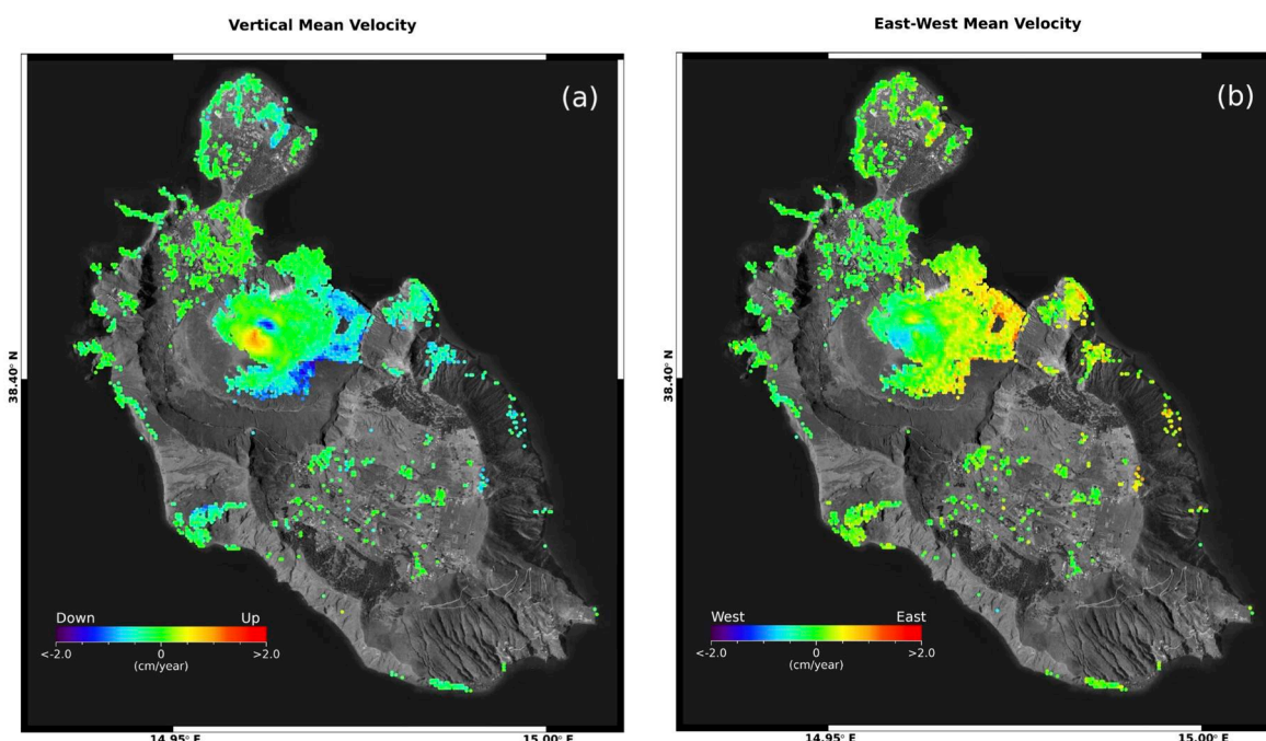
Figura 1. Vulcano: mappe delle componenti Verticale ed Est-Ovest della velocità media di deformazione relative al periodo 24 aprile 2015 – 14 maggio 2026 generate a partire da dati Sentinel-1. a) Componente Verticale. b) Componente Est-Ovest.
