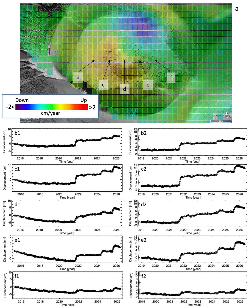
Figura 3. Vulcano – La Fossa: evoluzione temporale dello spostamento verticale per alcuni punti all'interno del cratere. a) mappa della componente Verticale della velocità di deformazione nel periodo 24 aprile 2015 – 14 maggio 2026. b1-f2) grafici dell'andamento temporale dello spostamento verticale per tutto il periodo analizzato (sinistra) e a partire da gennaio 2019 (destra), relativi ai punti identificati come b-f in Figura 3a.
