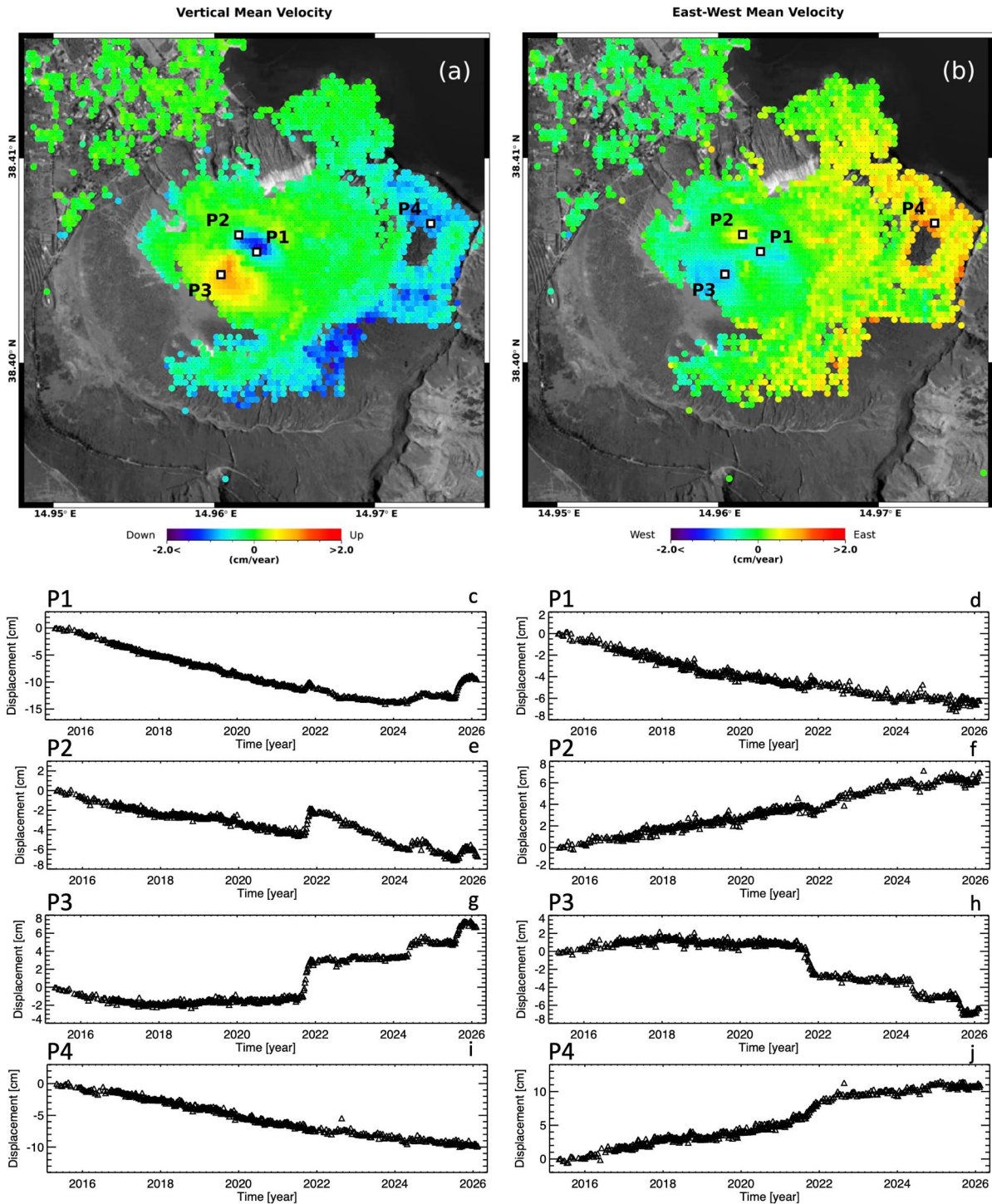
Figura 2. Vulcano – La Fossa: mappe delle componenti Verticale ed Est-Ovest della velocità media di deformazione relative al periodo 24 aprile 2015 – 13 febbraio 2026 generate a partire da dati Sentinel-1. a) Componente Verticale. b) Componente Est-Ovest. c-j) Andamento temporale della deformazione lungo la direzione Verticale (c)(e)(g)(i) ed Est-Ovest (d)(f)(h)(j) in corrispondenza di quattro punti identificati come P1, P2, P3 e P4 in (a)-(b).
