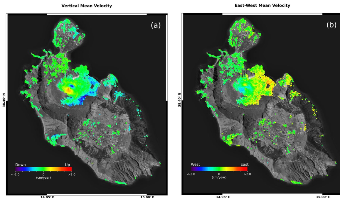
Figura 1. Vulcano: mappe delle componenti Verticale ed Est-Ovest della velocità media di deformazione relative al periodo 24 aprile 2015 – 13 febbraio 2026 generate a partire da dati Sentinel-1. a) Componente Verticale. b) Componente Est-Ovest.
