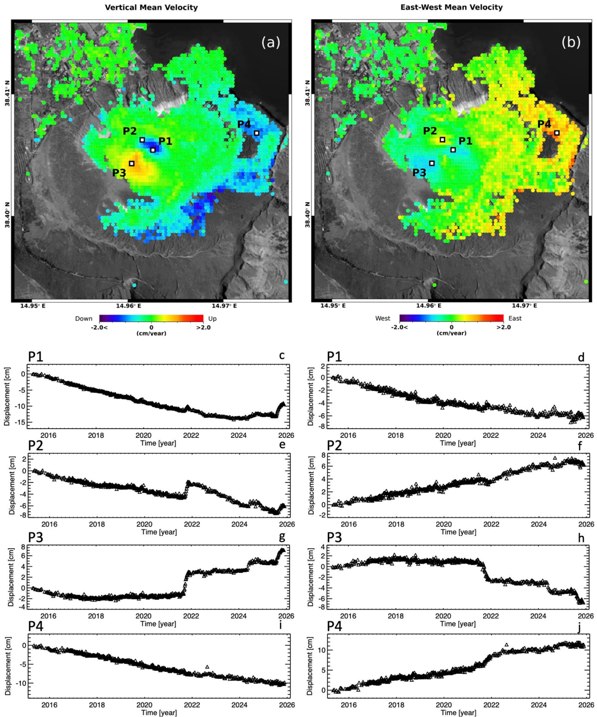
Figura 2. Vulcano – La Fossa: mappe delle componenti Verticale ed Est-Ovest della velocità media di deformazione relative al periodo 24 aprile 2015 – 27 novembre 2025 generate a partire da dati Sentinel-1. a) Componente Verticale. b) Componente Est-Ovest. c-j) Andamento temporale della deformazione lungo la direzione Verticale (c)(e)(g)(i) ed Est-Ovest (d)(f)(h)(j) in corrispondenza di quattro punti identificati come P1, P2, P3 e P4 in (a)-(b).
