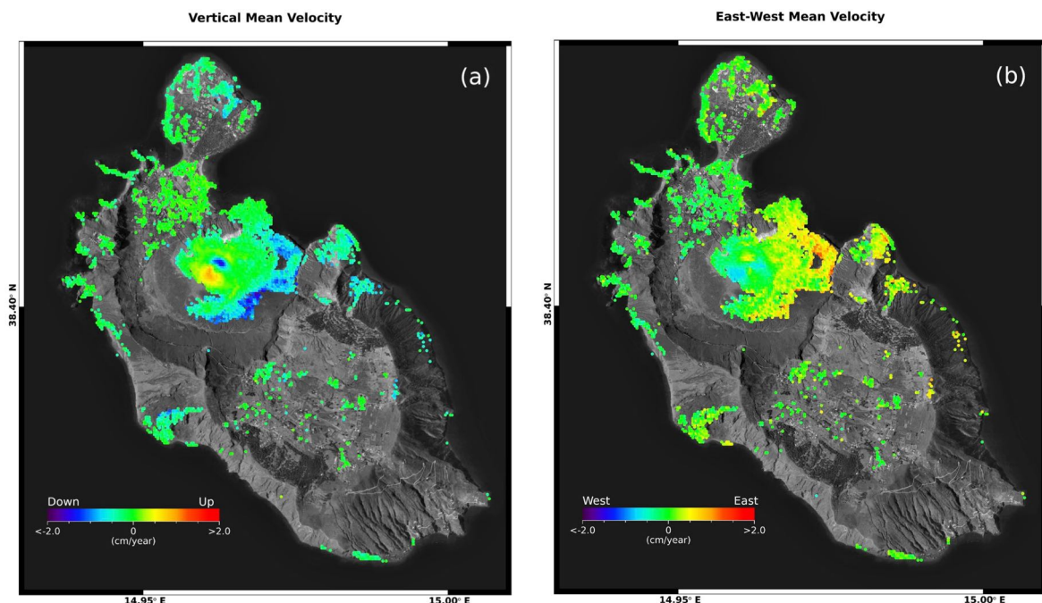
Figura 1. Vulcano: mappe delle componenti Verticale ed Est-Ovest della velocità media di deformazione relative al periodo 24 aprile 2015 – 27 novembre 2025 generate a partire da dati Sentinel-1. a) Componente Verticale. b) Componente Est-Ovest.
