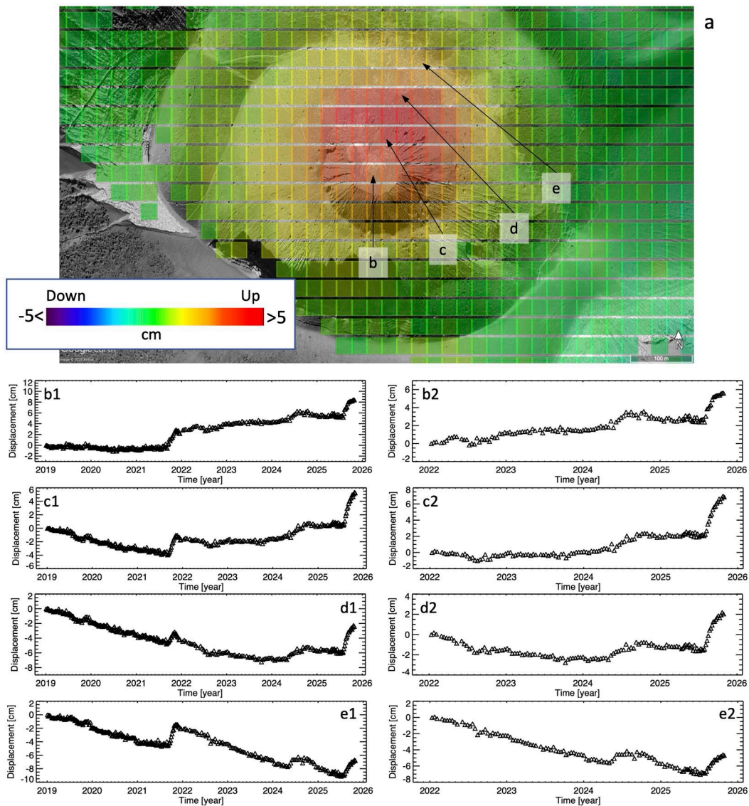
Figura 4. Vulcano – La Fossa: evoluzione temporale dello spostamento verticale per alcuni punti all'interno del cratere. a) mappa della componente Verticale dello spostamento del suolo nel periodo 30 luglio 2025 – 28 ottobre 2025. b1-e2) grafici dell'andamento temporale dello spostamento verticale da gennaio 2019 (sinistra) e da gennaio 2022 (destra), relativi ai punti identificati come b-e in Figura 4a.
