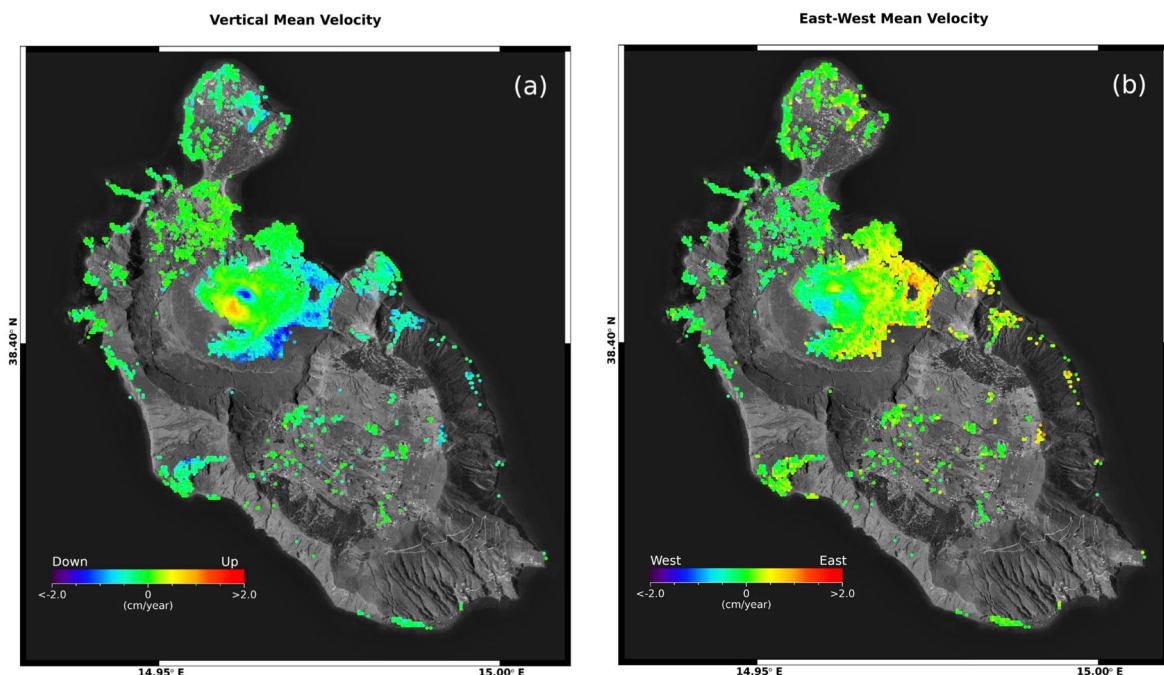
Figura 1. Vulcano: mappe delle componenti Verticale ed Est-Ovest della velocità media di deformazione relative al periodo 24 aprile 2015 – 28 ottobre 2025 generate a partire da dati Sentinel-1. a) Componente Verticale. b) Componente Est-Ovest.
