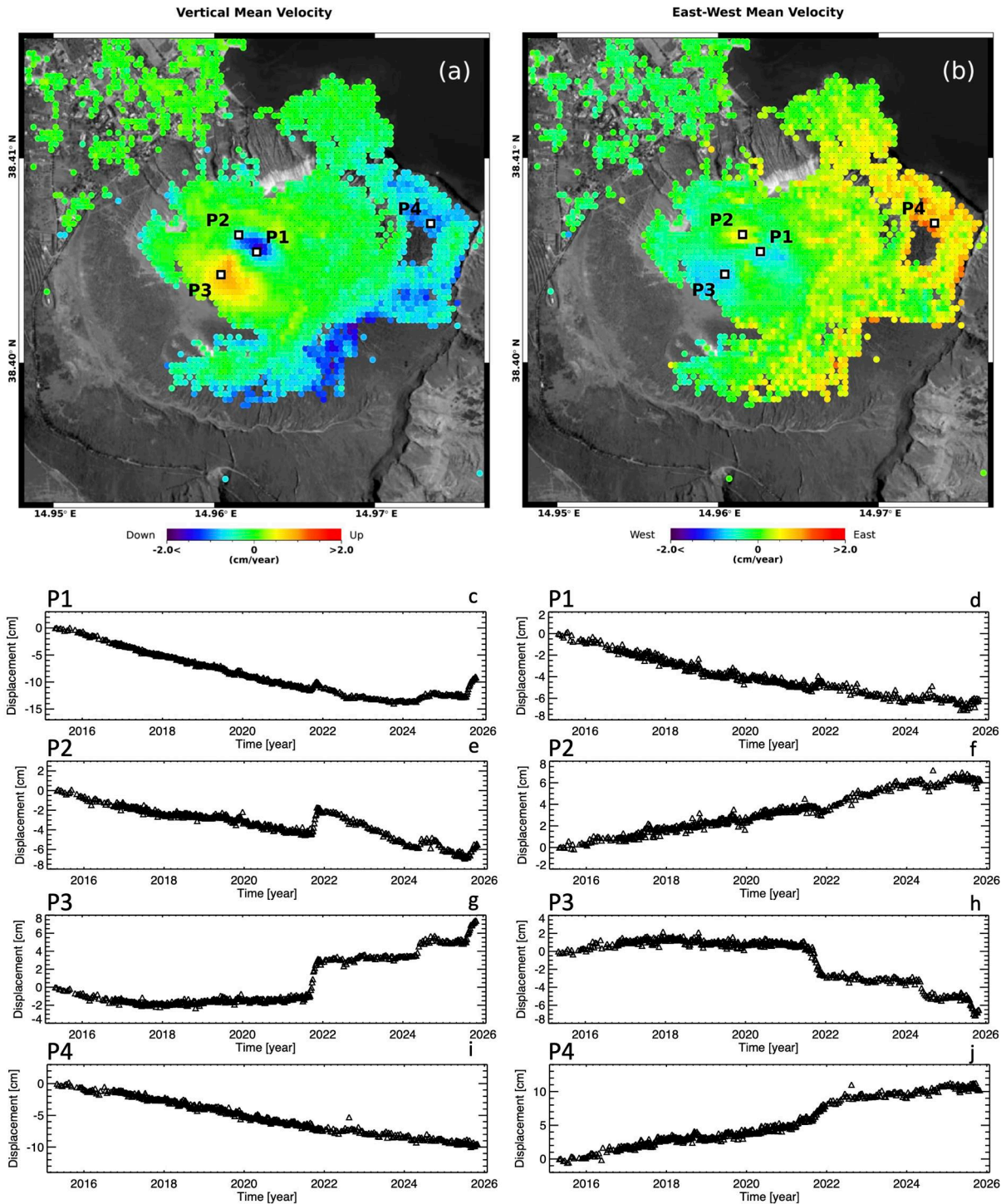
Figura 2. Vulcano – La Fossa: mappe delle componenti Verticale ed Est-Ovest della velocità media di deformazione relative al periodo 24 aprile 2015 – 28 ottobre 2025 generate a partire da dati Sentinel-1. a) Componente Verticale. b) Componente Est-Ovest. c-j) Andamento temporale della deformazione lungo la direzione Verticale (c)(e)(g)(i) ed Est-Ovest (d)(f)(h)(j) in corrispondenza di quattro punti identificati come P1, P2, P3 e P4 in (a)-(b).
