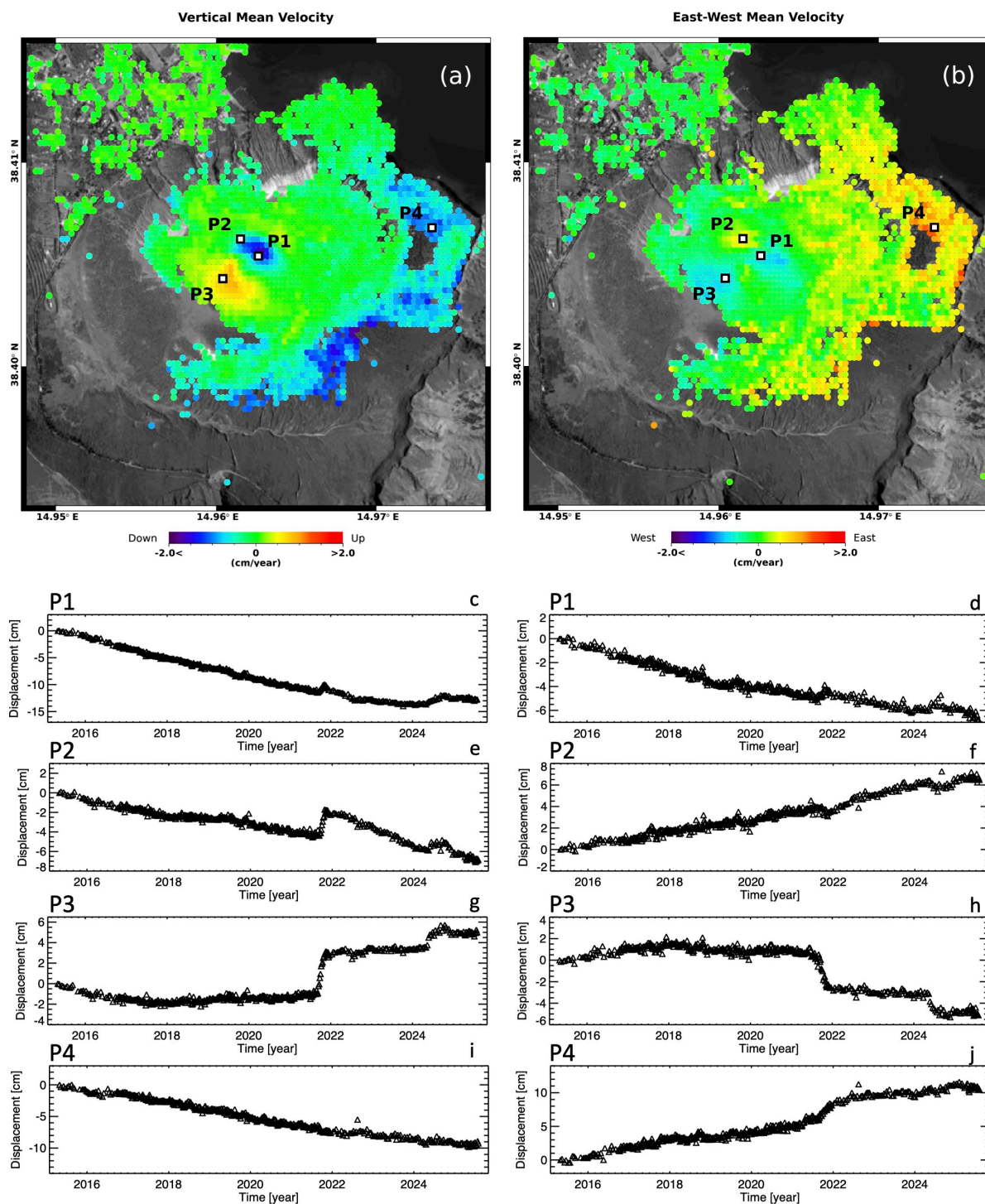
Figura 2. Vulcano – La Fossa: mappe delle componenti Verticale ed Est-Ovest della velocità media di deformazione relative al periodo 24 aprile 2015 – 30 luglio 2025 generate a partire da dati Sentinel-1. a) Componente Verticale. b) Componente Est-Ovest. c-j) Andamento temporale della deformazione lungo la direzione Verticale (c)(e)(g)(i) ed Est-Ovest (d)(f)(h)(j) in corrispondenza di quattro punti identificati come P1, P2, P3 e P4 in (a)-(b).
