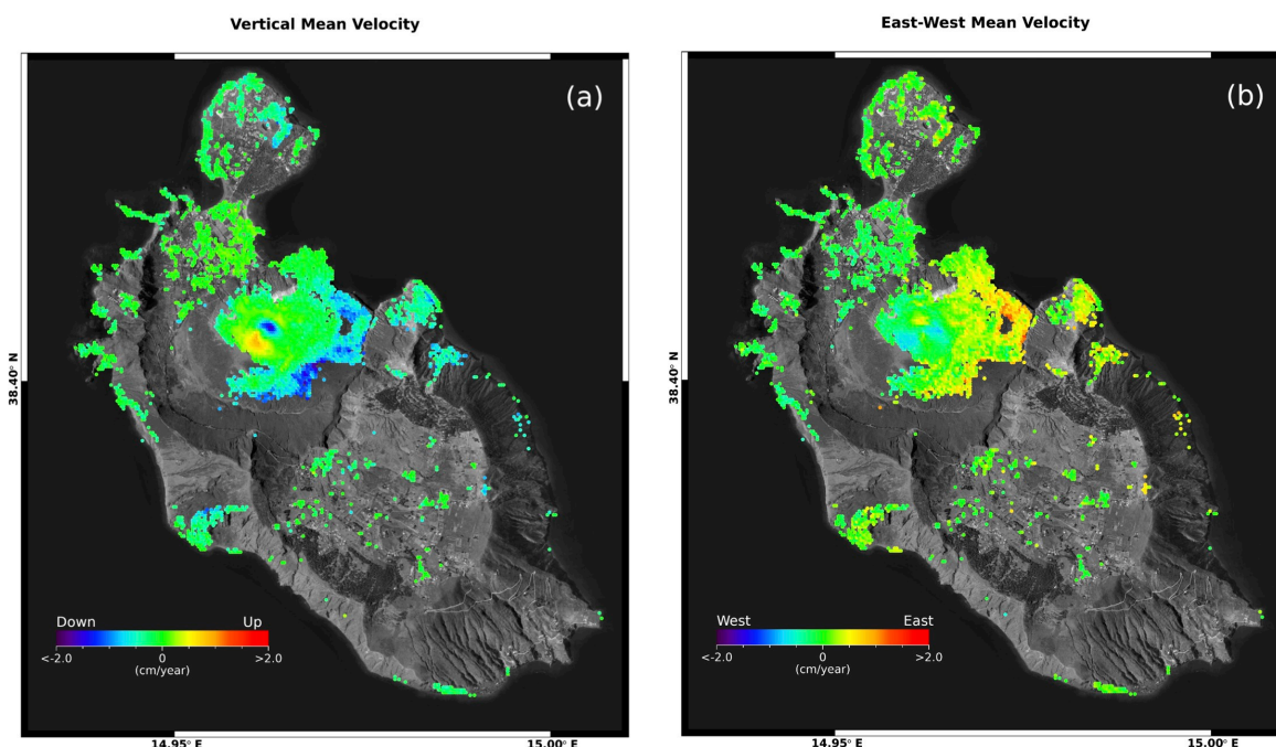
Figura 1. Vulcano: mappe delle componenti Verticale ed Est-Ovest della velocità media di deformazione relative al periodo 24 aprile 2015 – 30 luglio 2025 generate a partire da dati Sentinel-1. a) Componente Verticale. b) Componente Est-Ovest.
