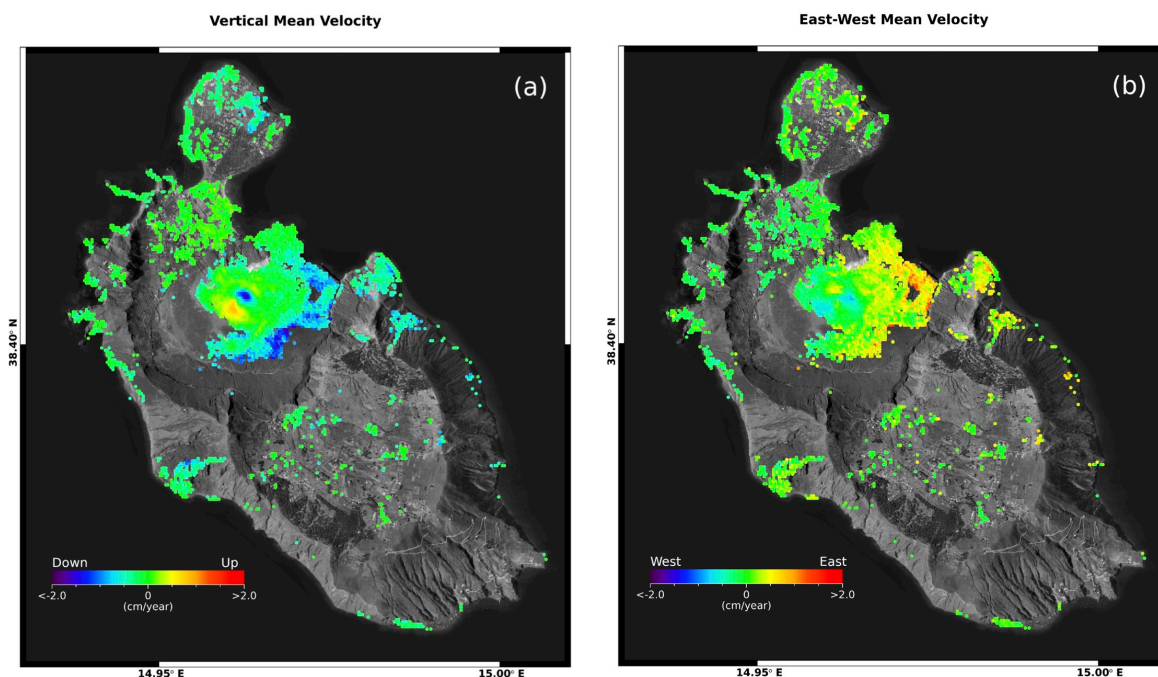
Figura 1. Vulcano: mappe delle componenti Verticale ed Est-Ovest della velocità media di deformazione relative al periodo 24 aprile 2015 – 1° maggio 2025 generate a partire da dati Sentinel-1. a) Componente Verticale. b) Componente Est-Ovest.
