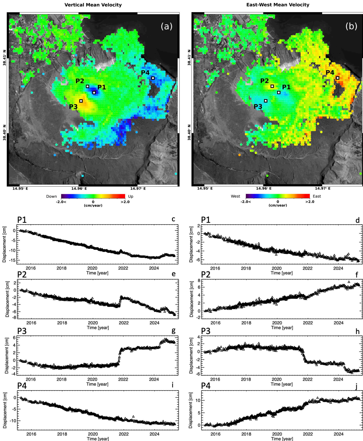
Figura 2. Vulcano – La Fossa: mappe delle componenti Verticale ed Est-Ovest della velocità media di deformazione relative al periodo 24 aprile 2015 – 1° maggio 2025 generate a partire da dati Sentinel-1. a) Componente Verticale. b) Componente Est-Ovest. c-j) Andamento temporale della deformazione lungo la direzione Verticale (c)(e)(g)(i) ed Est-Ovest (d)(f)(h)(j) in corrispondenza di quattro punti identificati come P1, P2, P3 e P4 in (a)-(b).
