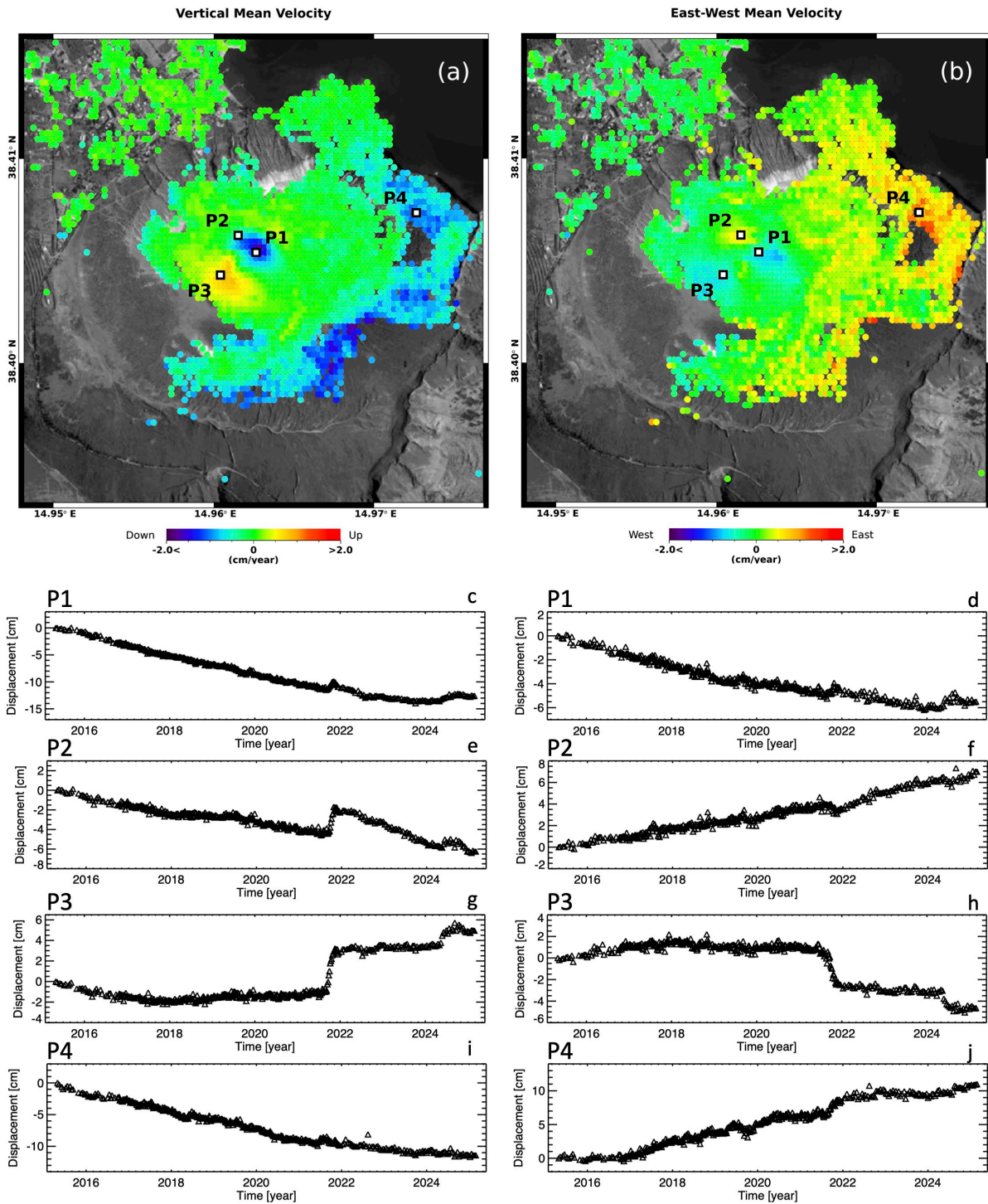
Figura 2. Vulcano – La Fossa: mappe delle componenti Verticale ed Est-Ovest della velocità media di deformazione relative al periodo 24 aprile 2015 – 2 marzo 2025 generate a partire da dati Sentinel-1. a) Componente Verticale. b) Componente Est-Ovest. c-j) Andamento temporale della deformazione lungo la direzione Verticale (c)(e)(g)(i) ed Est-Ovest (d)(f)(h)(j) in corrispondenza di quattro punti identificati come P1, P2, P3 e P4 in (a)-(b).
