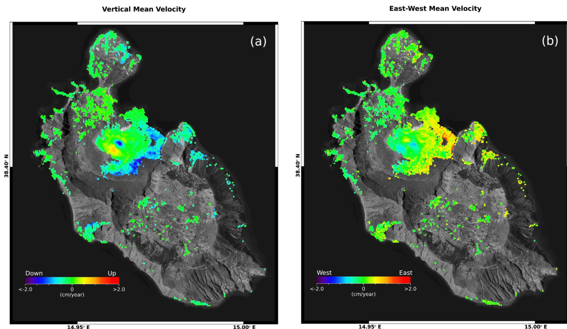
Figura 1. Vulcano: mappe delle componenti Verticale ed Est-Ovest della velocità media di deformazione relative al periodo 24 aprile 2015 – 2 marzo 2025 generate a partire da dati Sentinel-1. a) Componente Verticale. b) Componente Est-Ovest.
