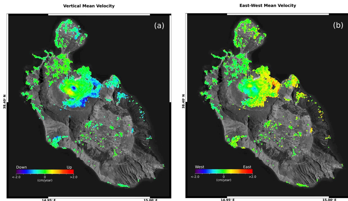
Figura 1. Vulcano: mappe delle componenti Verticale ed Est-Ovest della velocità media di deformazione relative al periodo 24 aprile 2015 – 29 giugno 2024 generate a partire da dati Sentinel-1. a) Componente Verticale. b) Componente Est-Ovest.
