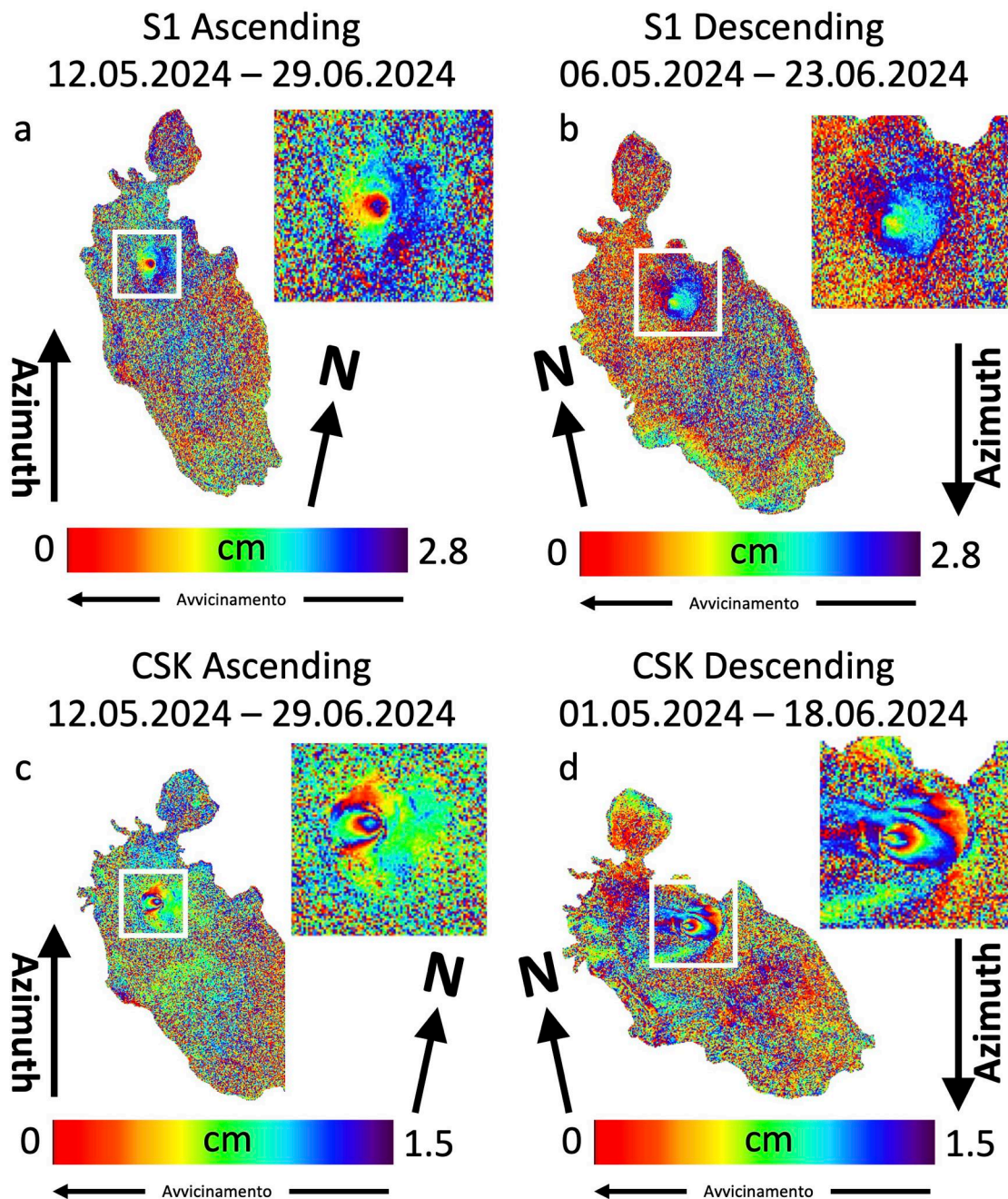
Figura 4. Interferogrammi differenziali, in geometria radar, generati a partire da dati acquisiti dai sensori (a-b) Sentinel-1 e (c-d) COSMO-SkyMed rispettivamente lungo orbite ascendenti e discendenti. Gli inserti mostrano una visione ravvicinata delle aree delimitate dai quadrati bianchi.
