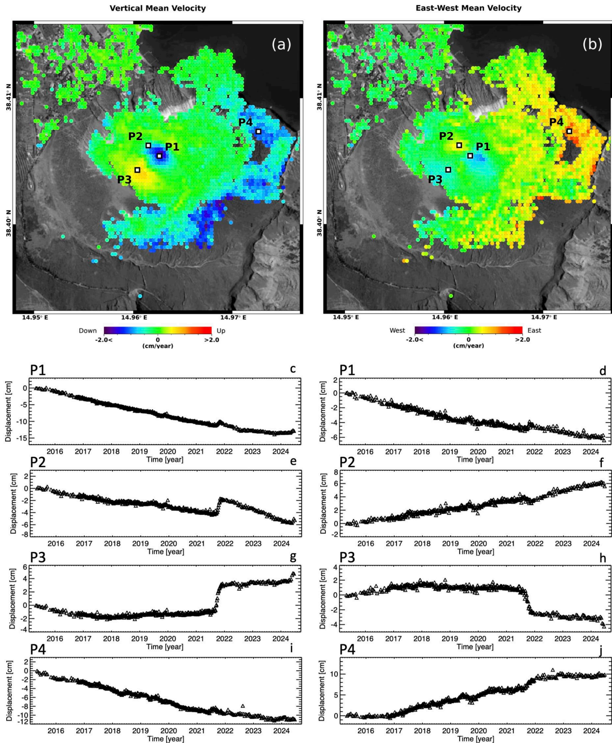
Figura 2. Vulcano – La Fossa: mappe delle componenti Verticale ed Est-Ovest della velocità media di deformazione relative al periodo 24 aprile 2015 – 29 giugno 2024 generate a partire da dati Sentinel-1. a) Componente Verticale. b) Componente Est-Ovest. c-j) Andamento temporale della deformazione lungo la direzione Verticale (c)(e)(g)(i) ed Est-Ovest (d)(f)(h)(j) in corrispondenza di quattro punti identificati come P1, P2, P3 e P4 in (a)-(b).
