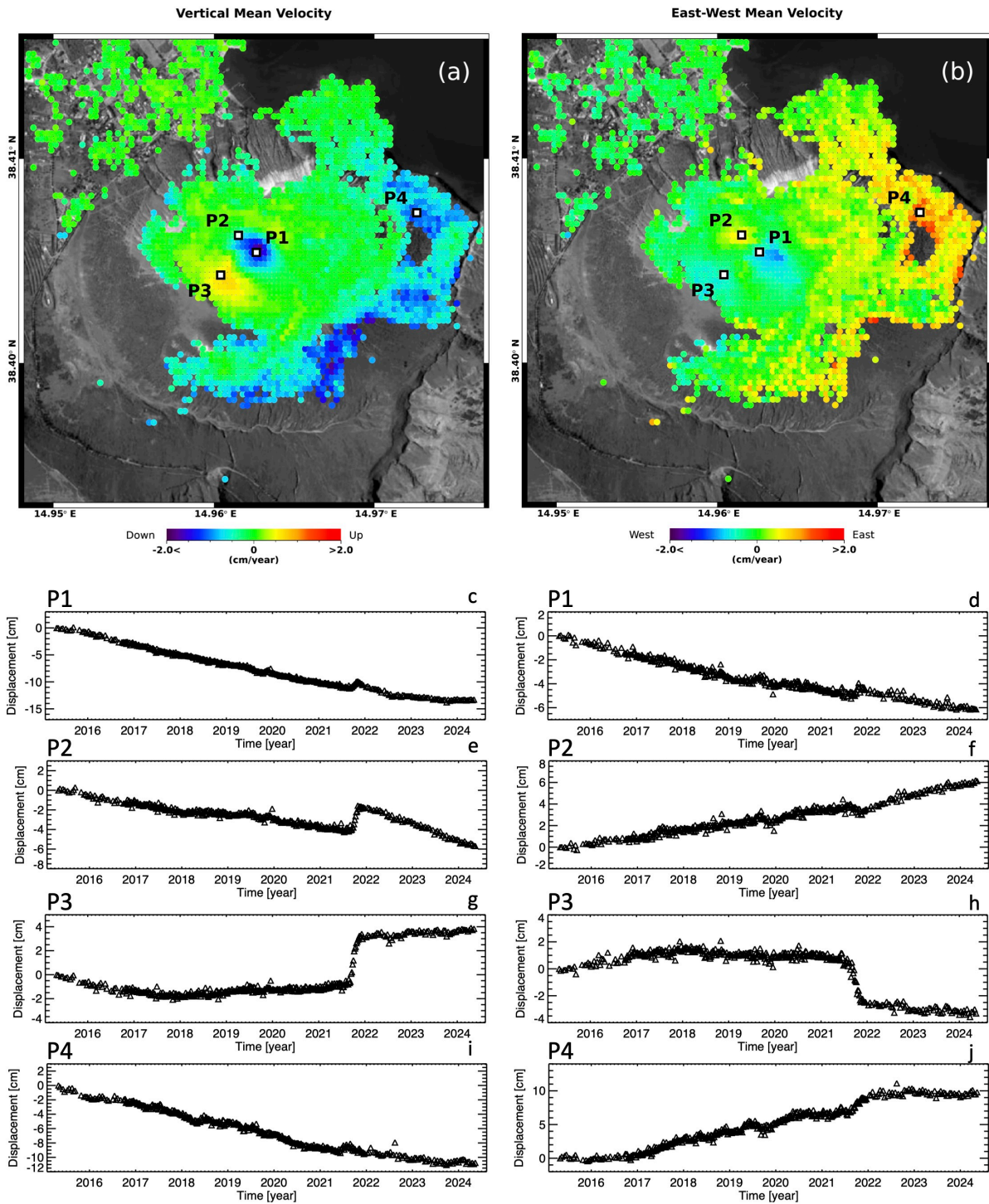
Figura 2. Vulcano – La Fossa: mappe delle componenti Verticale ed Est-Ovest della velocità media di deformazione relative al periodo 24 aprile 2015 – 24 maggio 2024 generate a partire da dati Sentinel-1. a) Componente Verticale. b) Componente Est-Ovest. c-j) Andamento temporale della deformazione lungo la direzione Verticale (c)(e)(g)(i) ed Est-Ovest (d)(f)(h)(j) in corrispondenza di quattro punti identificati come P1, P2, P3 e P4 in (a)-(b).
