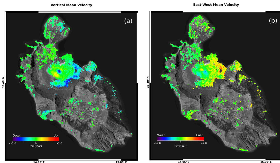
Figura 1. Vulcano: mappe delle componenti Verticale ed Est-Ovest della velocità media di deformazione relative al periodo 24 aprile 2015 – 24 maggio 2024 generate a partire da dati Sentinel-1. a) Componente Verticale. b) Componente Est-Ovest.
