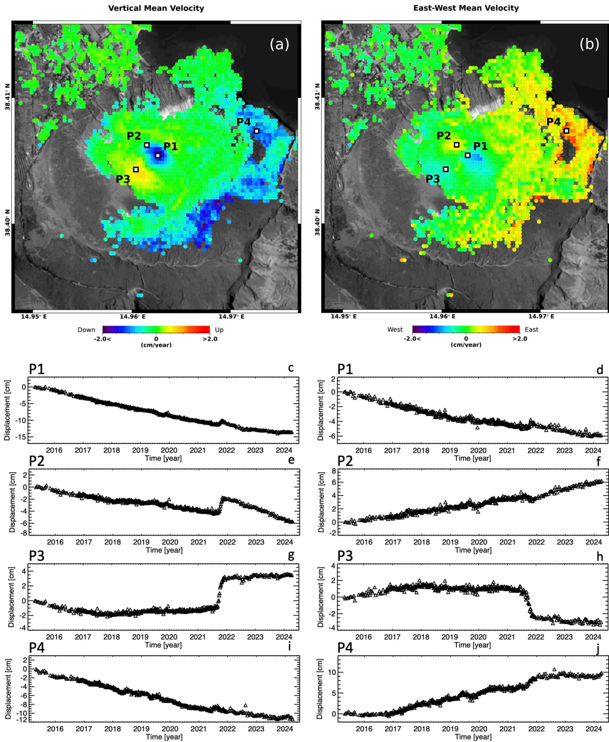
Figura 2. Vulcano – La Fossa: mappe delle componenti Verticale ed Est-Ovest della velocità media di deformazione relative al periodo 24 aprile 2015 – 18 aprile 2024 generate a partire da dati Sentinel-1. a) Componente Verticale. b) Componente Est-Ovest. c-j) Andamento temporale della deformazione lungo la direzione Verticale (c)(e)(g)(i) ed Est-Ovest (d)(f)(h)(j) in corrispondenza di quattro punti identificati come P1, P2, P3 e P4 in (a)-(b).
