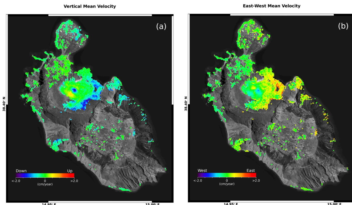
Figura 1. Vulcano: mappe delle componenti Verticale ed Est-Ovest della velocità media di deformazione relative al periodo 24 aprile 2015 – 18 aprile 2024 generate a partire da dati Sentinel-1. a) Componente Verticale. b) Componente Est-Ovest.
