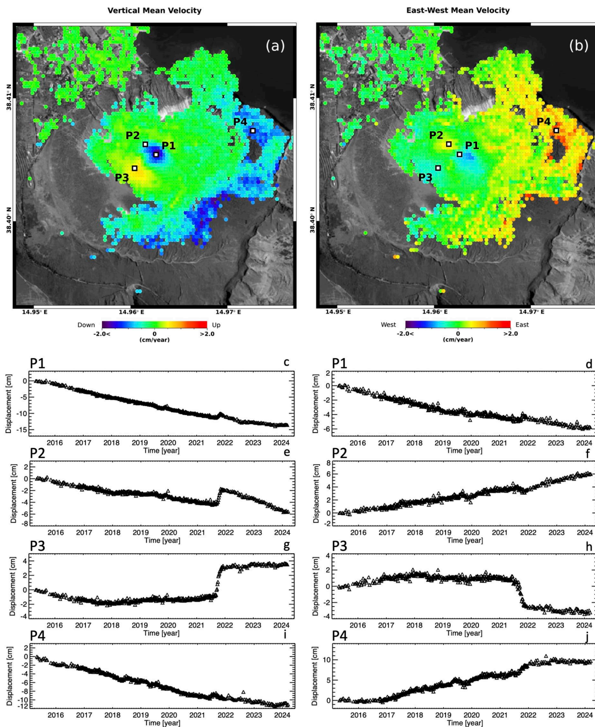
Figura 2. Vulcano – La Fossa: mappe delle componenti Verticale ed Est-Ovest della velocità media di deformazione relative al periodo 24 aprile 2015 – 19 marzo 2024 generate a partire da dati Sentinel-1. a) Componente Verticale. b) Componente Est-Ovest. c-j) Andamento temporale della deformazione lungo la direzione Verticale (c)(e)(g)(i) ed Est-Ovest (d)(f)(h)(j) in corrispondenza di quattro punti identificati come P1, P2, P3 e P4 in (a)-(b).
