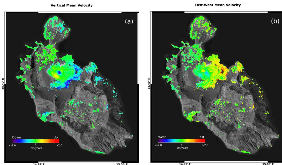
Figura 1. Vulcano: mappe delle componenti Verticale ed Est-Ovest della velocità media di deformazione relative al periodo 24 aprile 2015 – 19 marzo 2024 generate a partire da dati Sentinel-1. a) Componente Verticale. b) Componente Est-Ovest.
