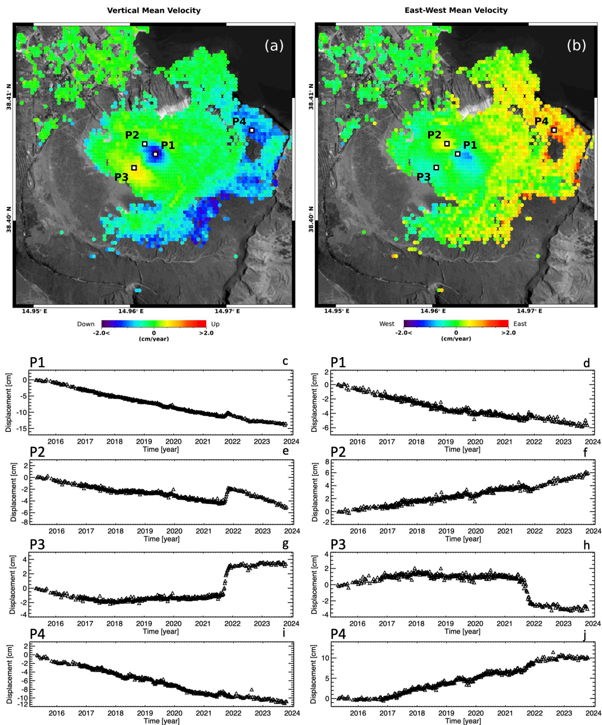
Figura 2. Vulcano – La Fossa: mappe delle componenti Verticale ed Est-Ovest della velocità media di deformazione relative al periodo 24 aprile 2015 – 2 novembre 2023 generate a partire da dati Sentinel-1. a) Componente Verticale. b) Componente Est-Ovest. c-j) Andamento temporale della deformazione lungo la direzione Verticale (c)(e)(g)(i) ed Est-Ovest (d)(f)(h)(j) in corrispondenza di quattro punti identificati come P1, P2, P3 e P4 in (a)-(b).
