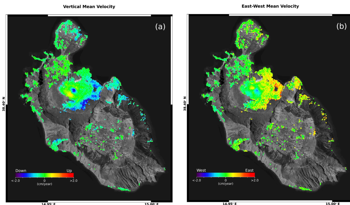
Figura 1. Vulcano: mappe delle componenti Verticale ed Est-Ovest della velocità media di deformazione relative al periodo 24 aprile 2015 – 2 novembre 2023 generate a partire da dati Sentinel-1. a) Componente Verticale. b) Componente Est-Ovest.
