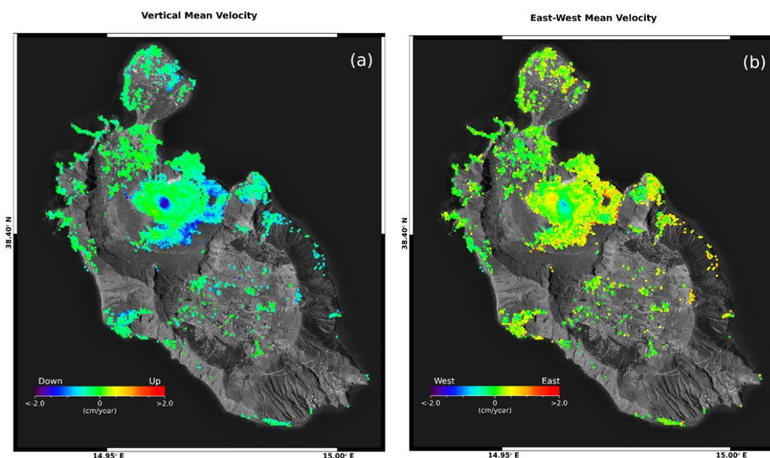
Figura 1. Vulcano: mappe delle componenti Verticale ed Est-Ovest della velocità media di deformazione relative al periodo 24 aprile 2015 – 24 novembre 2021 generate a partire da dati Sentinel-1. a) Componente Verticale. b) Componente Est-Ovest.
