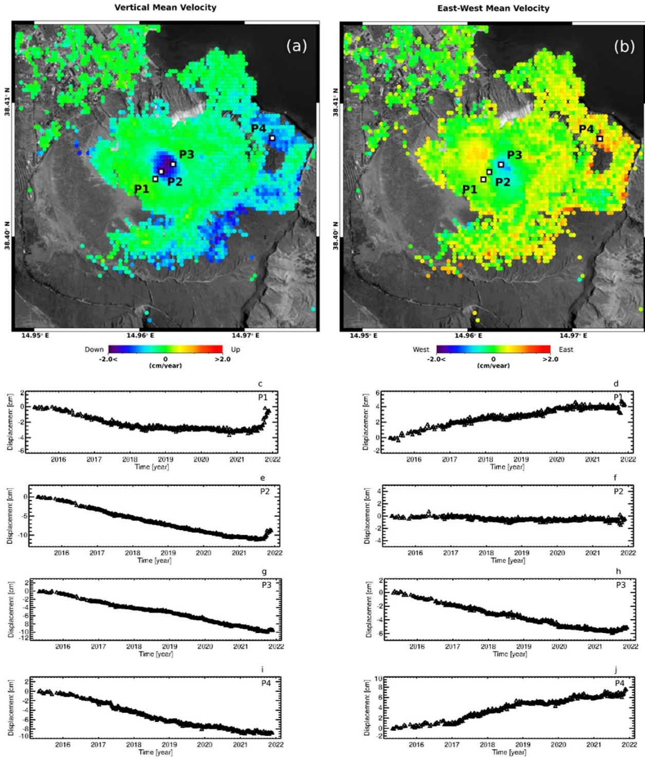
Figura 2. Vulcano – La Fossa: mappe delle componenti Verticale ed Est-Ovest della velocità media di deformazione relative al periodo 24 aprile 2015 – 24 novembre 2021 generate a partire da dati Sentinel-1. a) Componente Verticale. b) Componente Est-Ovest. c-j) Andamento temporale della deformazione lungo la direzione Verticale (c)(e)(g)(i) ed Est-Ovest (d)(f)(h)(j) in corrispondenza di quattro punti identificati come P1, P2, P3 e P4 in (a)-(b).
