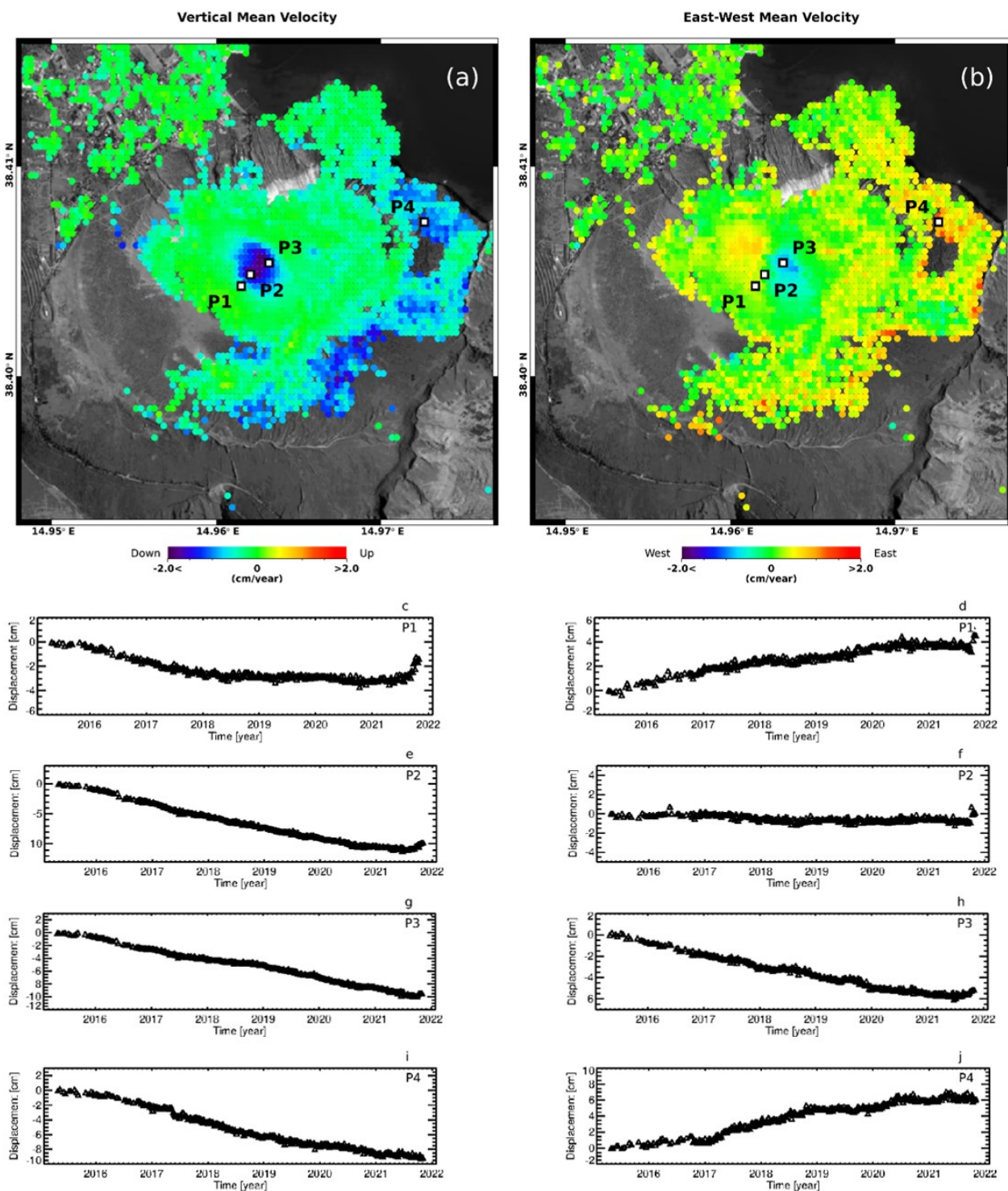
Figura 2. Vulcano – La Fossa: mappe delle componenti Verticale ed Est-Ovest della velocità media di deformazione relative al periodo 24 aprile 2015 – 31 ottobre 2021 generate a partire da dati Sentinel-1. a) Componente Verticale. b) Componente Est-Ovest. c-j) Andamento temporale della deformazione lungo la direzione Verticale (c)(e)(g)(i) ed Est-Ovest (d)(f)(h)(j) in corrispondenza di quattro punti identificati come P1, P2, P3 e P4 in (a)-(b).
