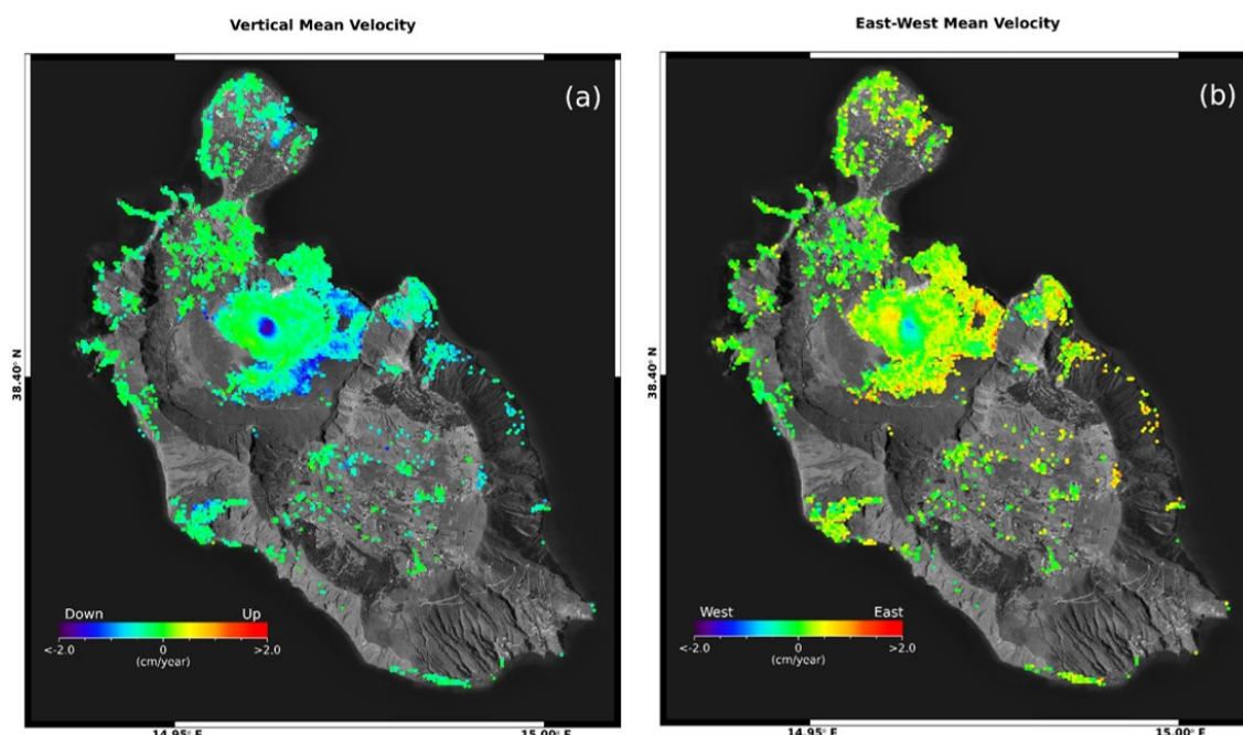
Figura 1. Vulcano: mappe delle componenti Verticale ed Est-Ovest della velocità media di deformazione relative al periodo 24 aprile 2015 – 31 ottobre 2021 generate a partire da dati Sentinel-1. a) Componente Verticale. b) Componente Est-Ovest.
