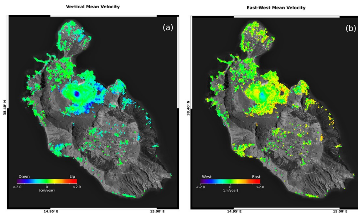
Figura 1. Vulcano: mappe delle componenti Verticale ed Est-Ovest della velocità media di deformazione relative al periodo 24 aprile 2015 – 25 settembre 2021 generate a partire da dati Sentinel-1. a) Componente Verticale. b) Componente Est-Ovest.
