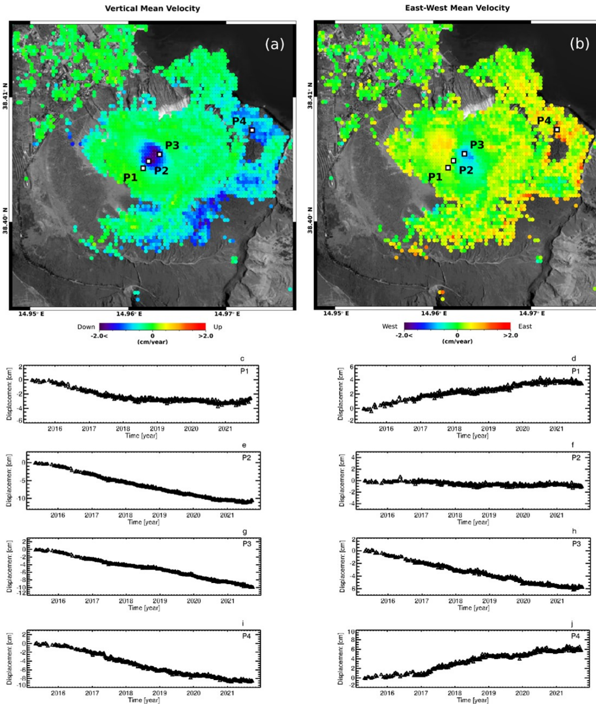
Figura 2. Vulcano – La Fossa: mappe delle componenti Verticale ed Est-Ovest della velocità media di deformazione relative al periodo 24 aprile 2015 – 25 settembre 2021 generate a partire da dati Sentinel-1. a) Componente Verticale. b) Componente Est-Ovest. c-j) Andamento temporale della deformazione lungo la direzione Verticale (c)(e)(g)(i) ed Est-Ovest (d)(f)(h)(j) in corrispondenza di quattro punti identificati come P1, P2, P3 e P4 in (a)-(b).
