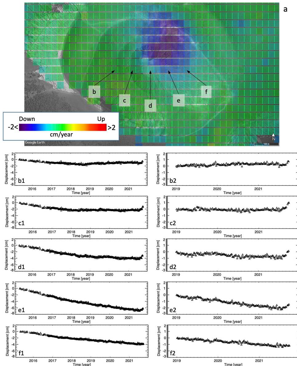
Figura 3. Vulcano – La Fossa: evoluzione temporale dello spostamento per alcuni punti all'interno del cratere. a) mappa della componente Verticale della velocità media di deformazione relativa al periodo 24 aprile 2015 – 25 settembre 2021. b1-f2) grafici dell'andamento temporale dello spostamento (per tutto il periodo analizzato e a partire da gennaio 2019) relativo ai punti identificati come b-f in Figura 3.
